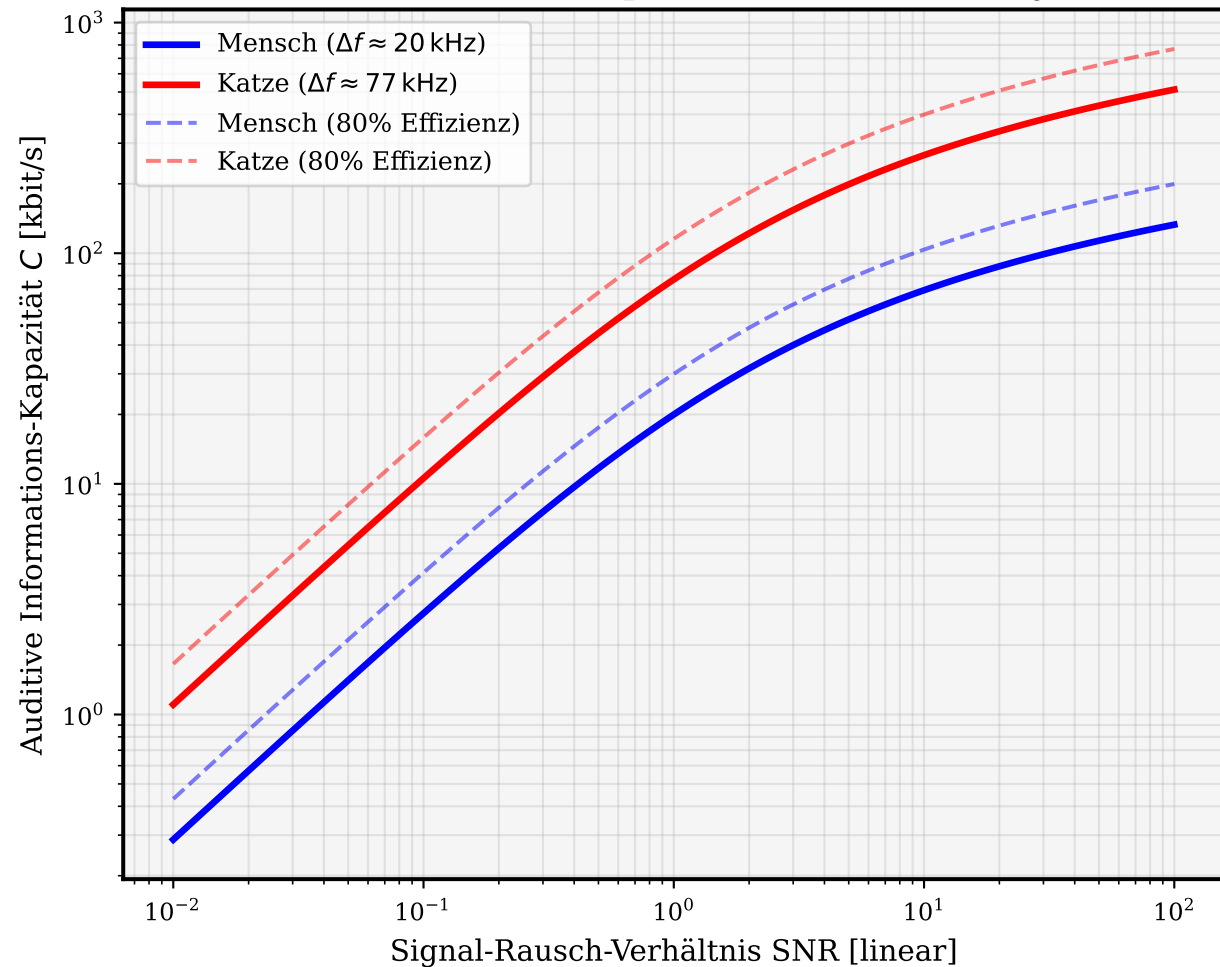
Shannon-Informationskapazität des auditiven Systems
