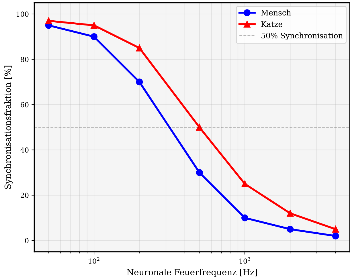
Neuronale Synchronisation und Phasen-Locking
