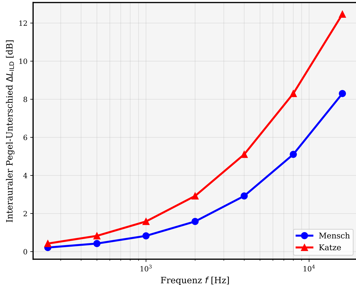
ILD als Funktion der Frequenz (90° Azimut)
