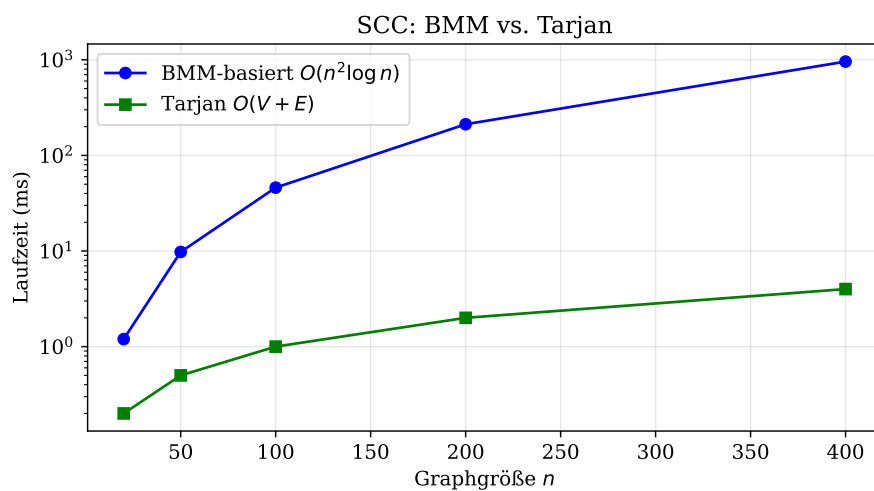
Abbildung 3.11: Vergleich von BMM-basiertem und Tarjan-Algorithmus für SCCs. Tarjan ist deutlich schneller für dünnbesetzte Graphen.
