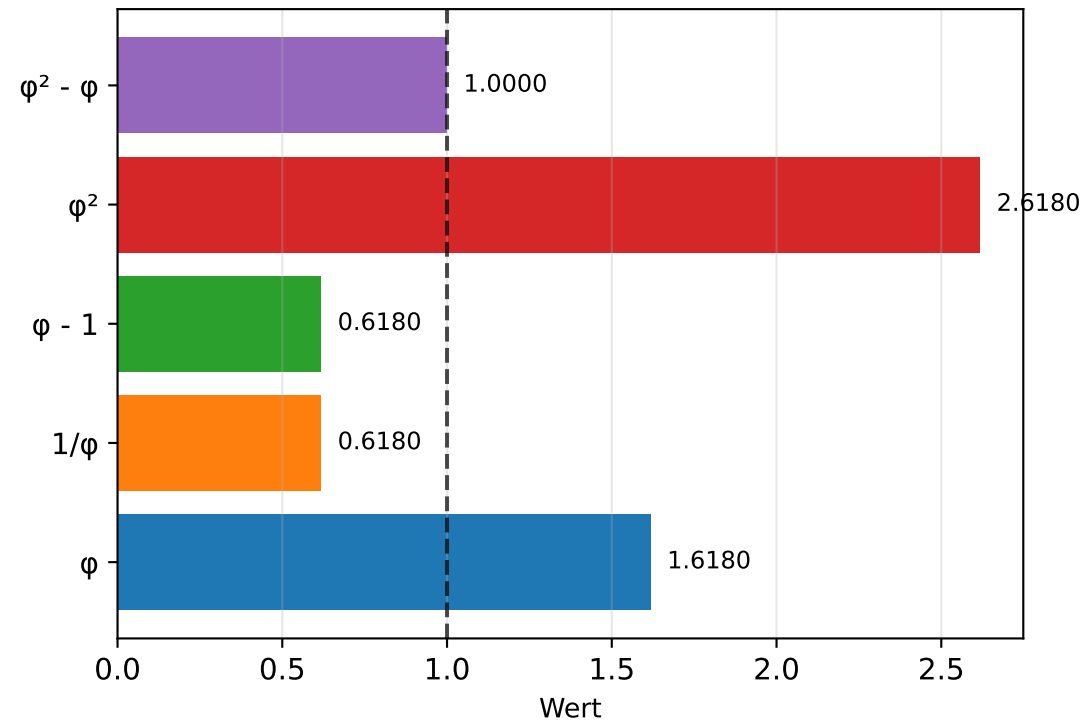
Algebraische Eigenschaften des Goldenen Schnitts
