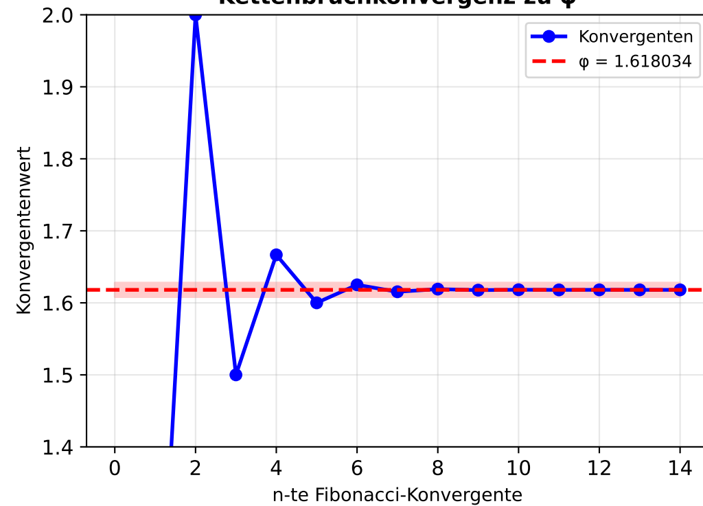
Kettenbruchkonvergenz zu \varphi
