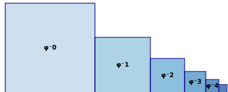
Selbstähnliche Zerlegung: \varphi = 1 + 1/\varphi
