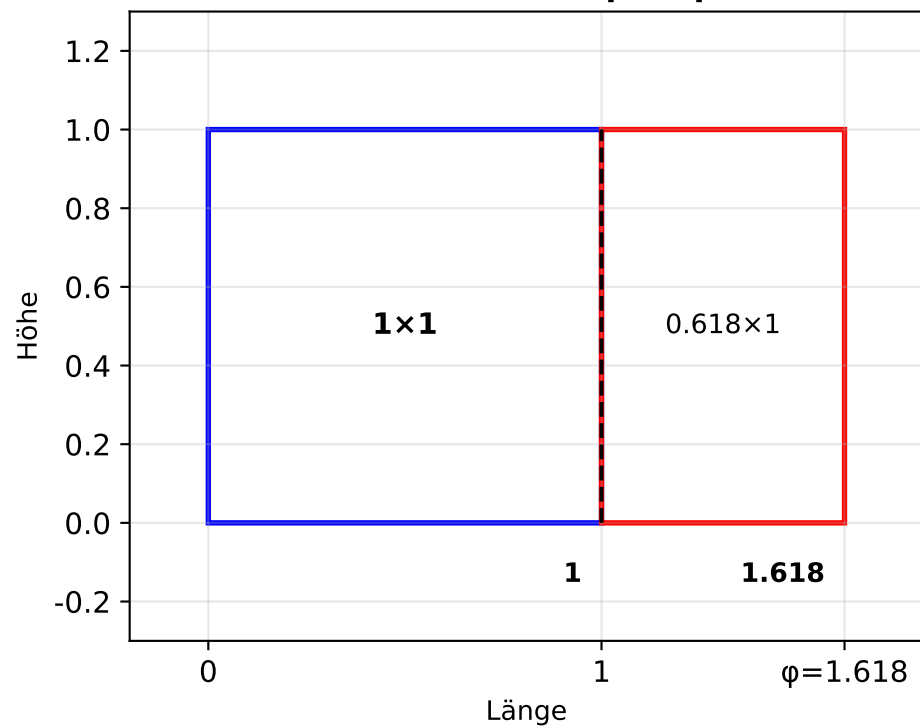
Goldener Schnitt: \varphi^2 = \varphi + 1
