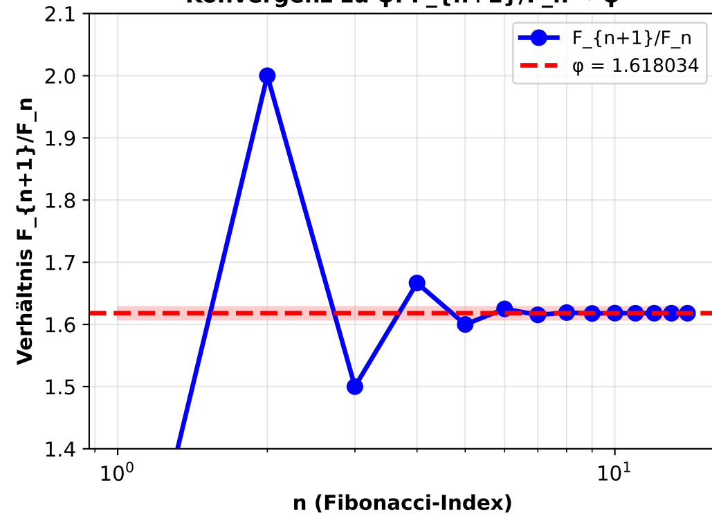
Konvergenz zu \varphi : F_{n+1}/F_n \rightarrow \varphi
