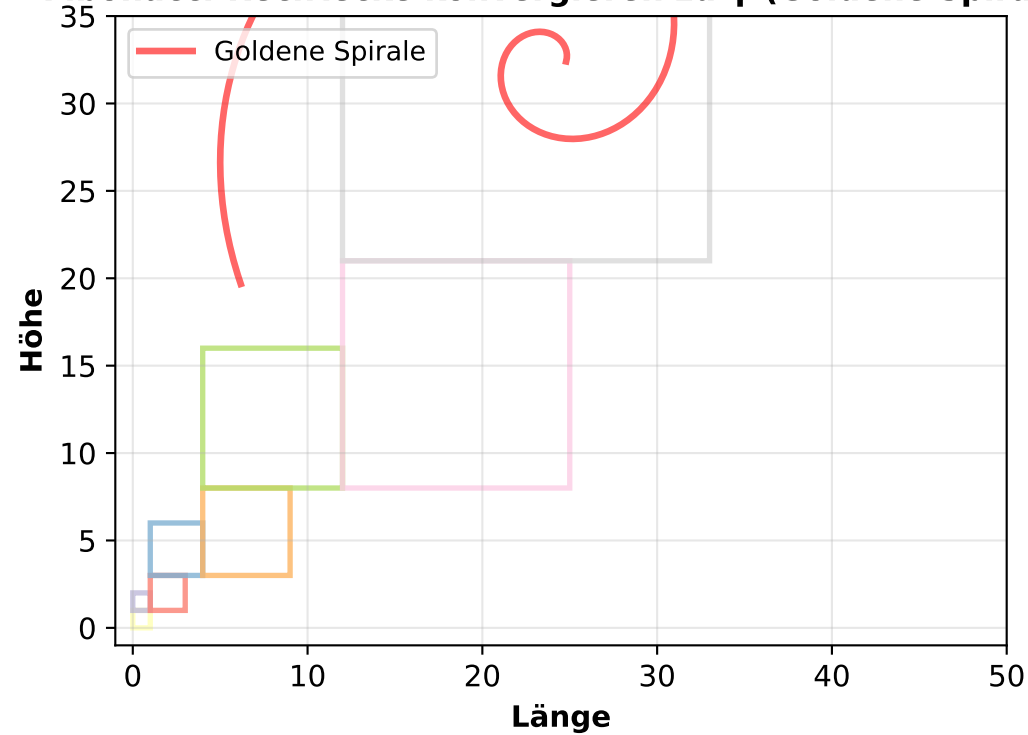
Fibonacci-Rechtecke konvergieren zu \varphi (Goldene Spirale)
