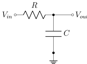
Abbildung 1: Der Tiefpassfilter
