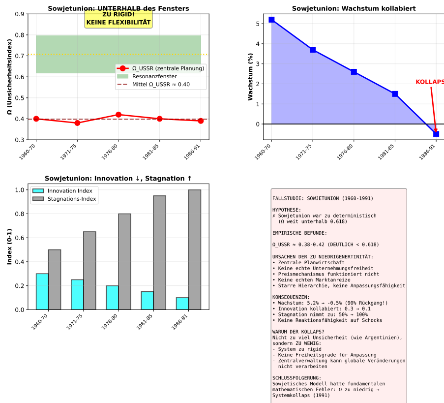
Abbildung 9: Der Plot veranschaulicht die modellierte Unterdeterminierung der sowjetischen Wirtschaft im Zeitraum 1960 bis 1991.
