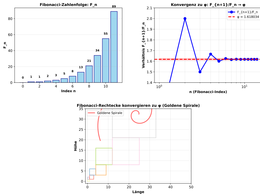
Abbildung 5: Der Plot verbindet das Wachstum der Fibonacci-Zahlen, die Quotientenkonvergenz zu \phi und die zugehörige Rechteckkonstruktion.
