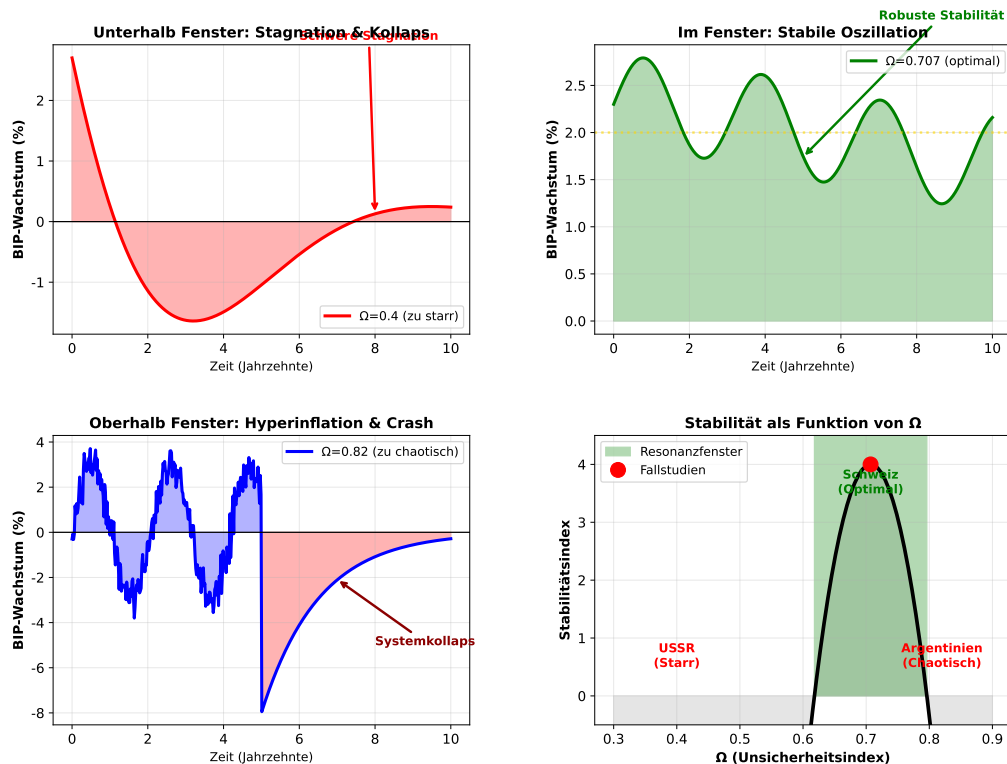
Abbildung 13: Der Plot vergleicht die modellierte Entwicklung unterhalb, innerhalb und oberhalb des Resonanzfensters.
