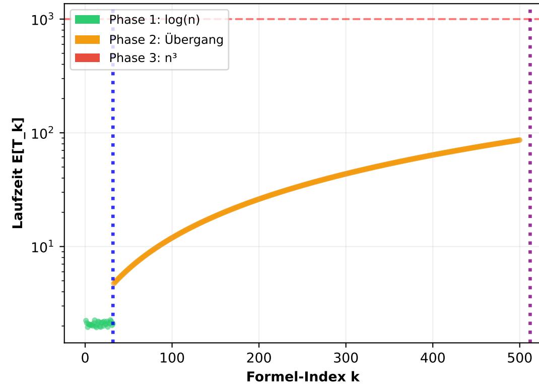
n = 14: Phasenstruktur
