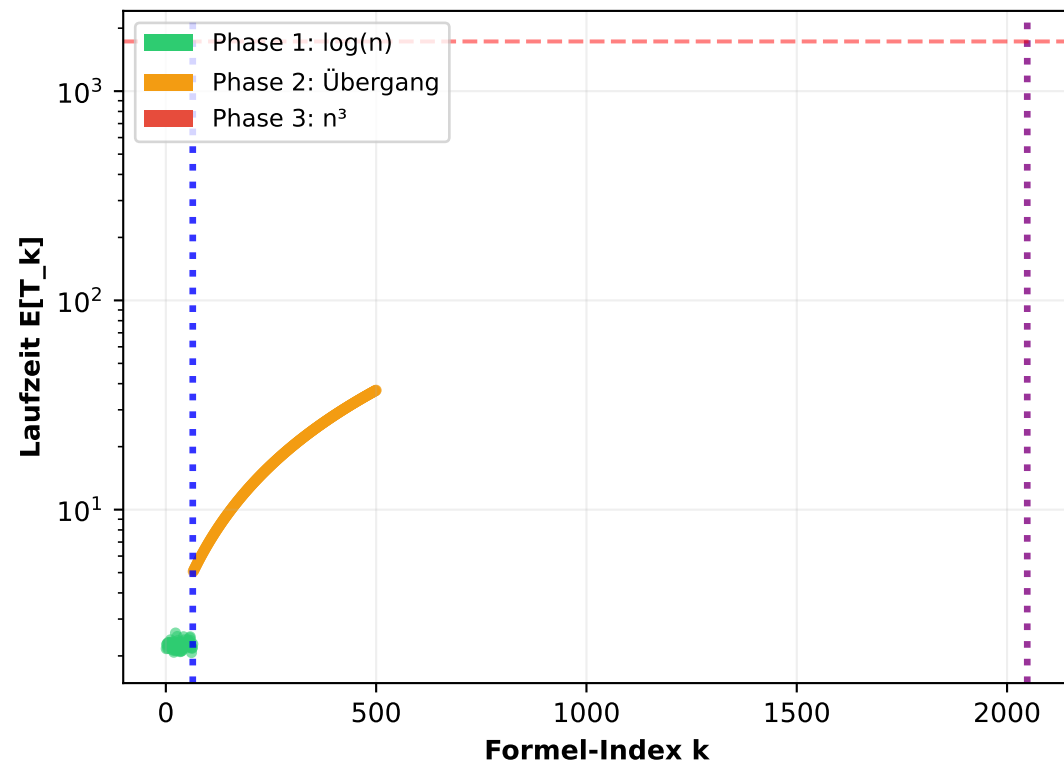
n = 12: Phasenstruktur
