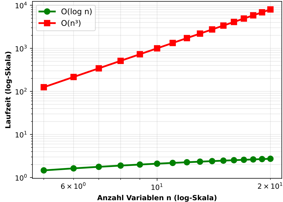
Wachstums-Raten beim Erhöhen von n
