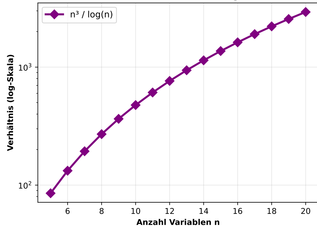
Dominanz von n^3 über \log(n)
