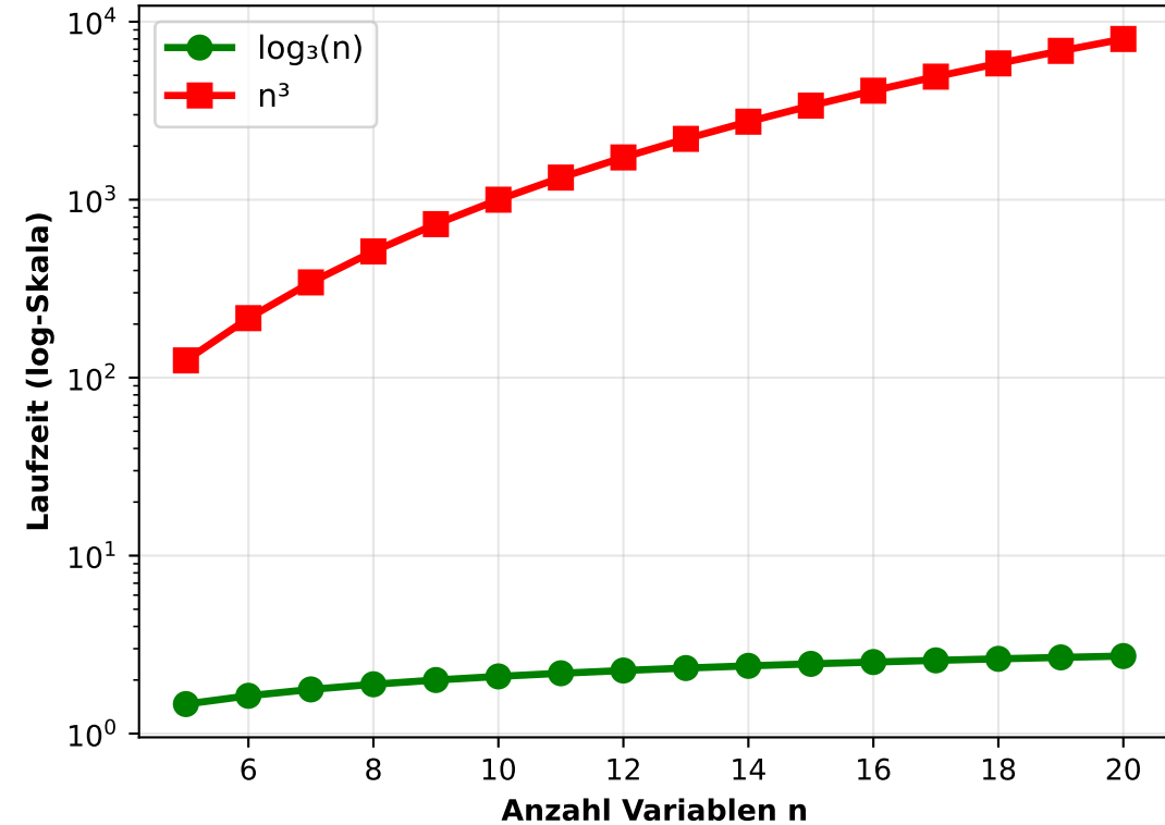
Dominanz von n^3 über \log(n)
