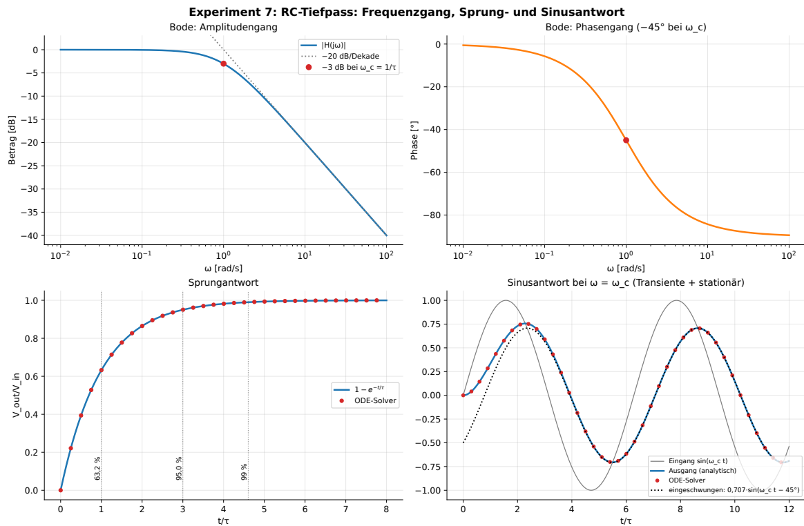
Abbildung 8: Die vier Teilgrafiken zeigen Betrag und Phase des Frequenzgangs sowie Sprung- und Sinusantwort des RC-Tiefpasses.
