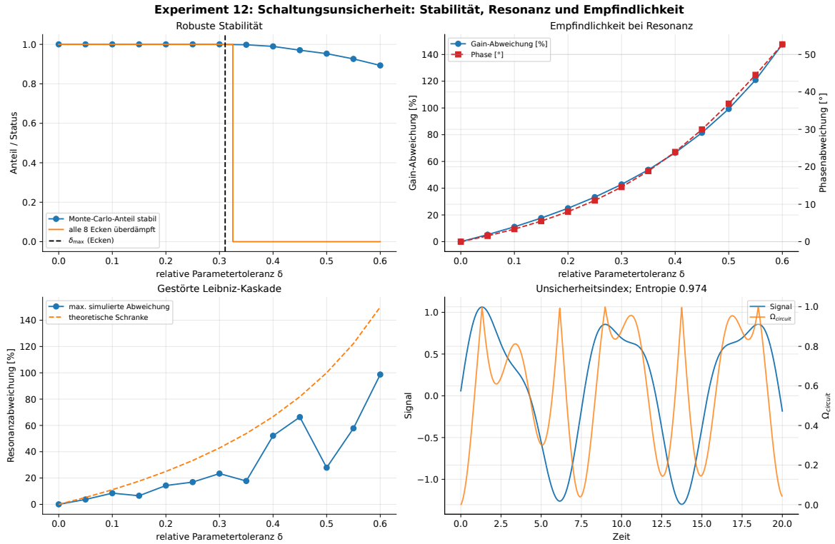
Abbildung 13: Oben links sind Monte-Carlo-Stabilitätsanteil und Eckpunktprüfung dargestellt; oben rechts die Gain- und Phasenabweichung. Unten links stehen simulierte Resonanzabweichungen ihrer Schranke gegenüber, unten rechts das synthetische Signal und der daraus berechnete Index \Omega_{\text{circuit}} .
