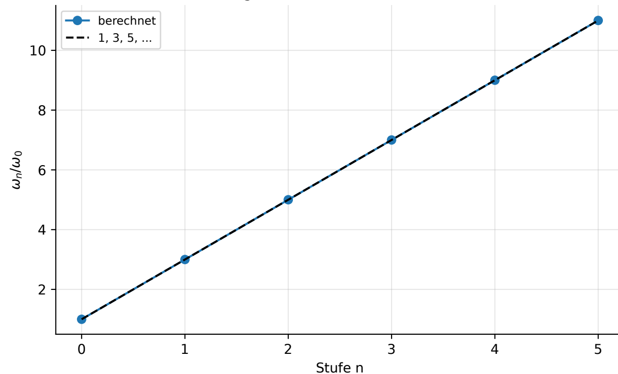
Vergleich der RC-Kaskaden
