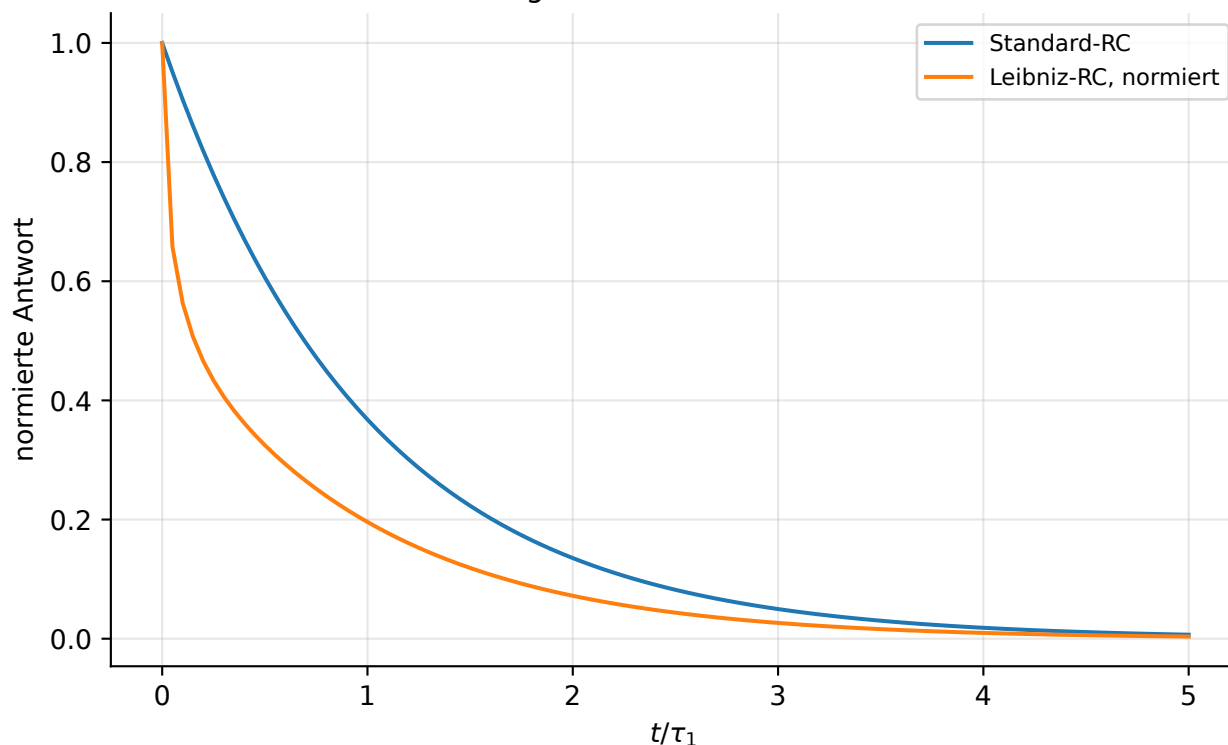
Vergleich der RC-Kaskaden
