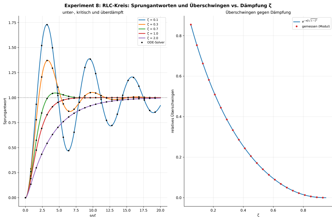
Abbildung 9: Die beiden Teilgrafiken vergleichen RLC-Sprungantworten und das relative Überschwüngen als Funktion des Dämpfungsgrades.
