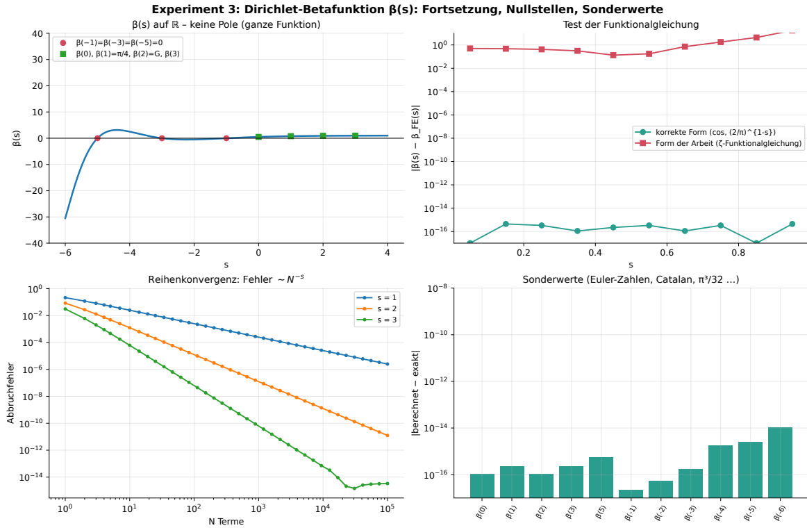
Abbildung 6: Die vier Teilgrafiken untersuchen Funktionswerte, Funktionalgleichung, Reihenkonvergenz und Sonderwerte von \beta(s) .
