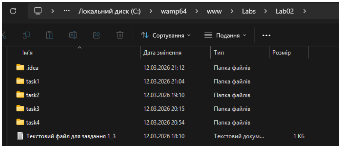
Рис. 4. Задання 1.3.
