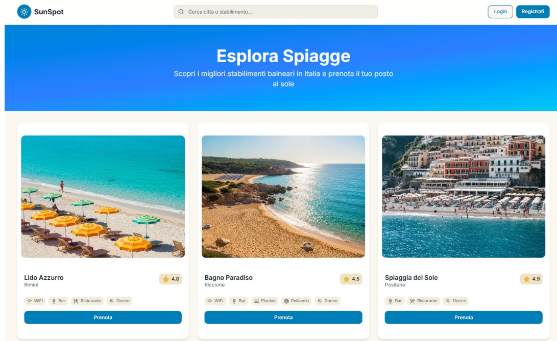
Figura 14: Esplora Spiagge - Desktop (UC-04): Interfaccia desktop per la ricerca nel catalogo. La vista interroga in sola lettura (CQRS tramite la BeachCatalogQuery ) il database, mostrando esclusivamente le spiagge in stato ATTIVO ed esponendo la valutazione media.
