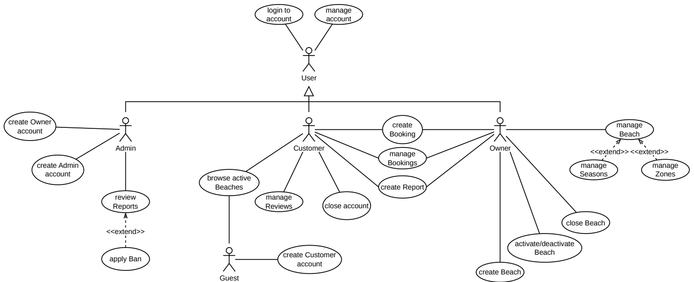
Figura 1: Diagramma degli Use Cases
