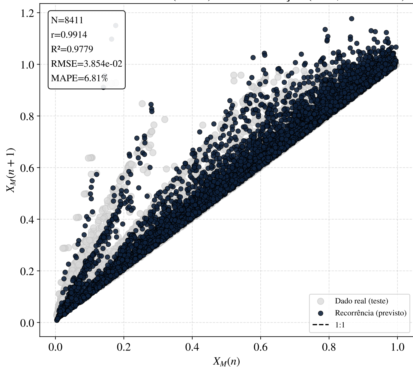
Recorrência Ancorada (esfera) — sem correção (teste, 528 curvas)
