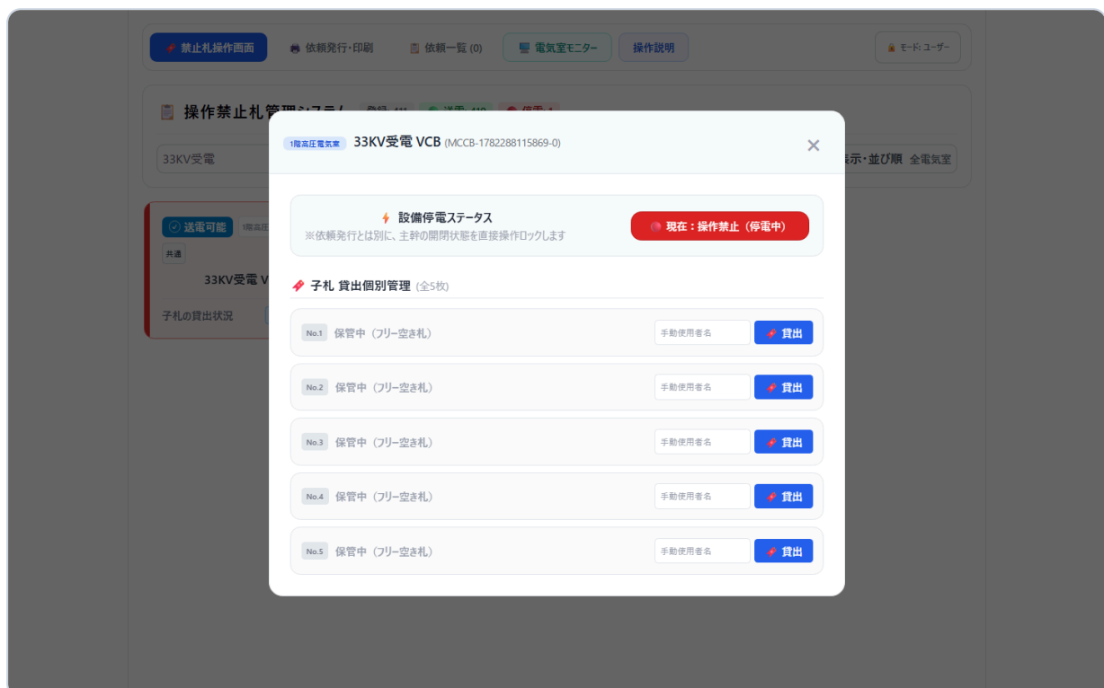
実画面 3: 送電直前に設備名・子札数・停電中状態を確認
