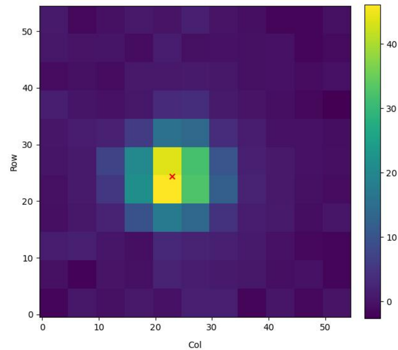
SNR Flux
