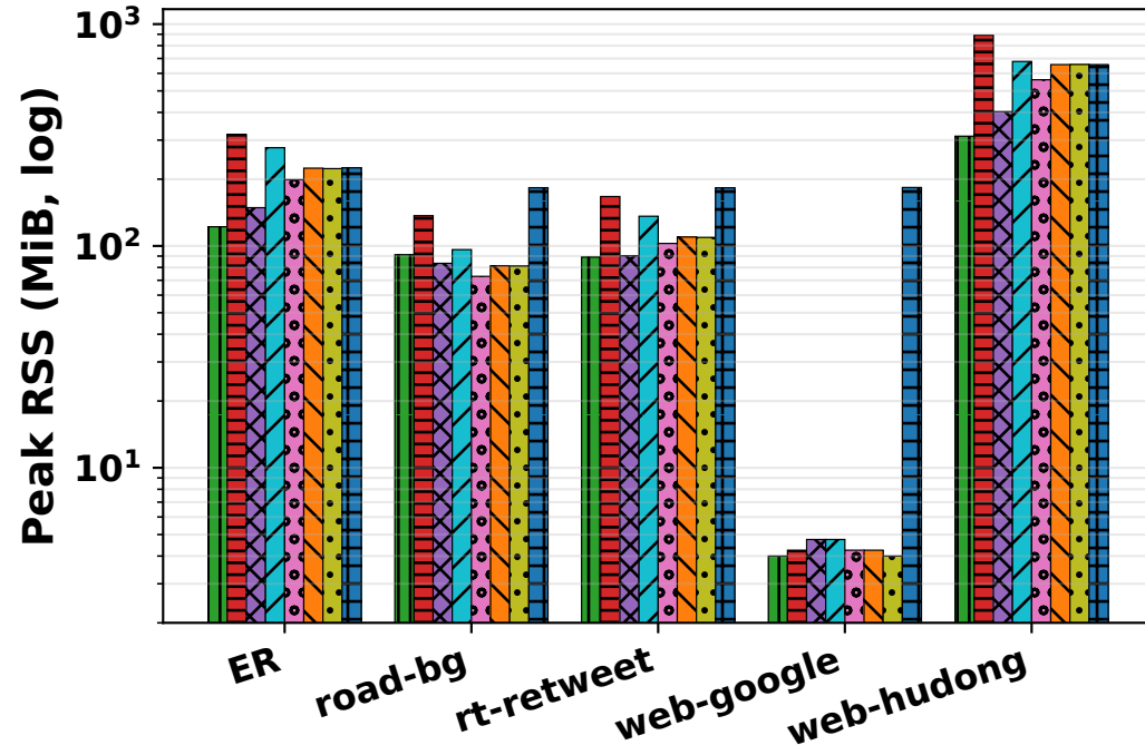
(d) pagerank
