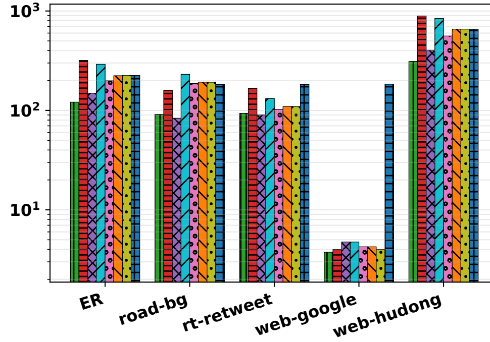
(e) sssp
