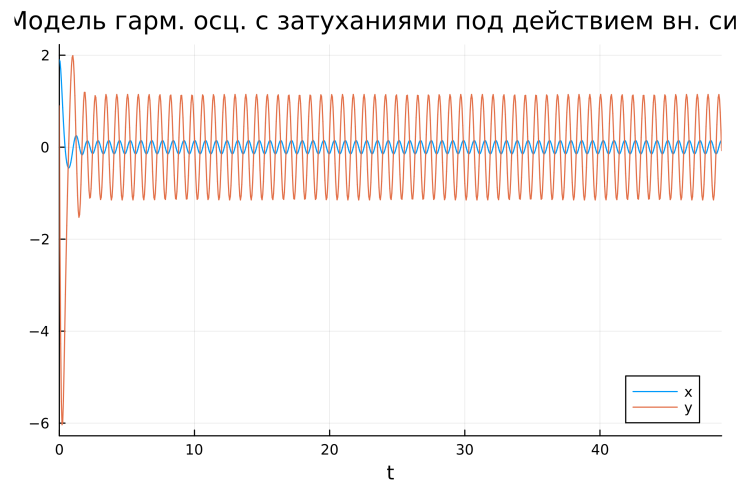
Рис. 4.9: Колебания гармонического осциллятора для третьего случая на Julia
