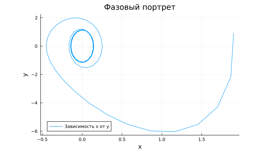
Рис. 4.10: Фазовый портрет колебаний гармонического осциллятора для третьего случая на Julia
