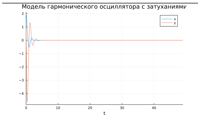
Рис. 4.5: Колебания гармонического осциллятора для второго случая на Julia
