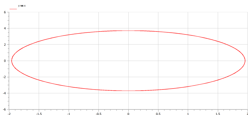
Рис. 4.4: Фазовый портрет колебаний гармонического осциллятора для первого случая на OpenModelica
