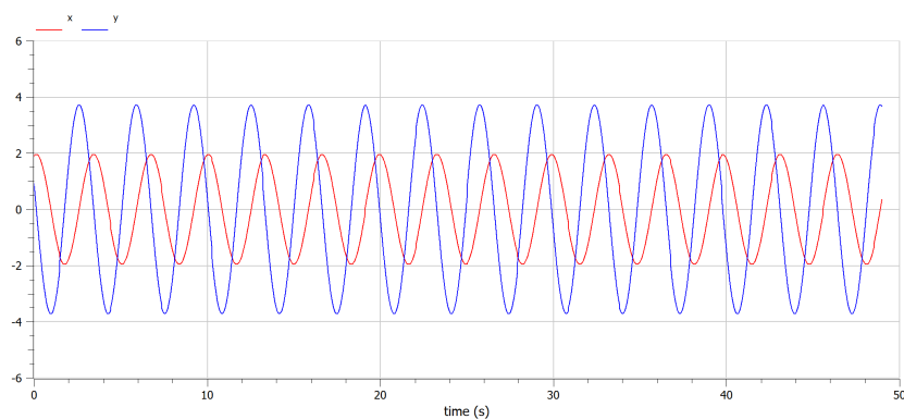
Рис. 4.3: Колебания гармонического осциллятора для первого случая на OpenModelica
