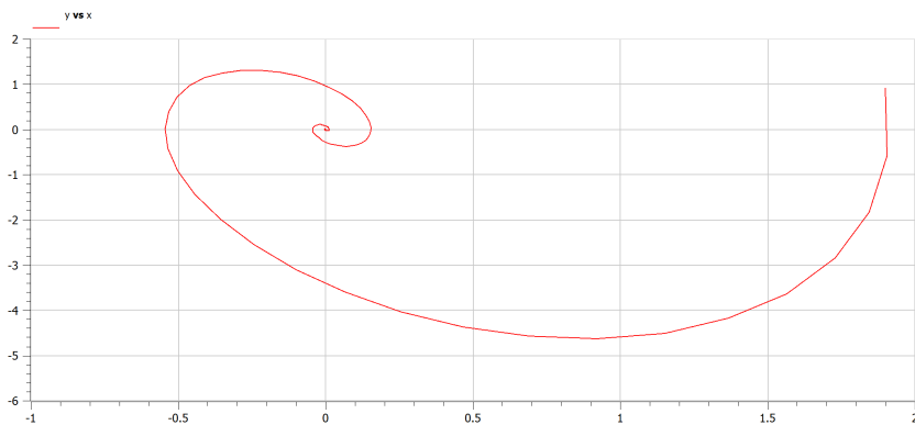
Рис. 4.8: Фазовый портрет колебаний гармонического осциллятора для второго случая на OpenModelica
