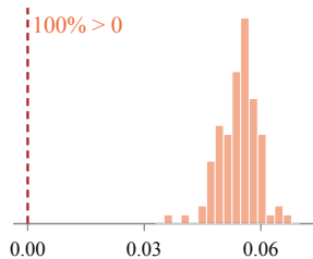
AIME 2024
