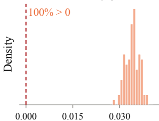
AIME 2025
