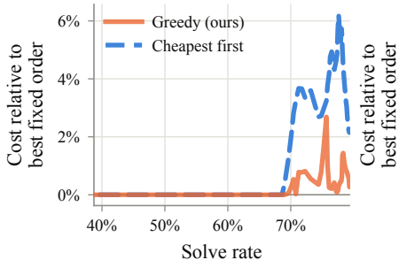
LiveCodeBench
