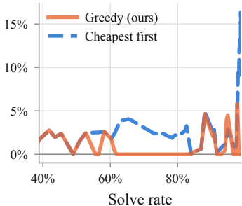
Terminal-Bench 2.0
