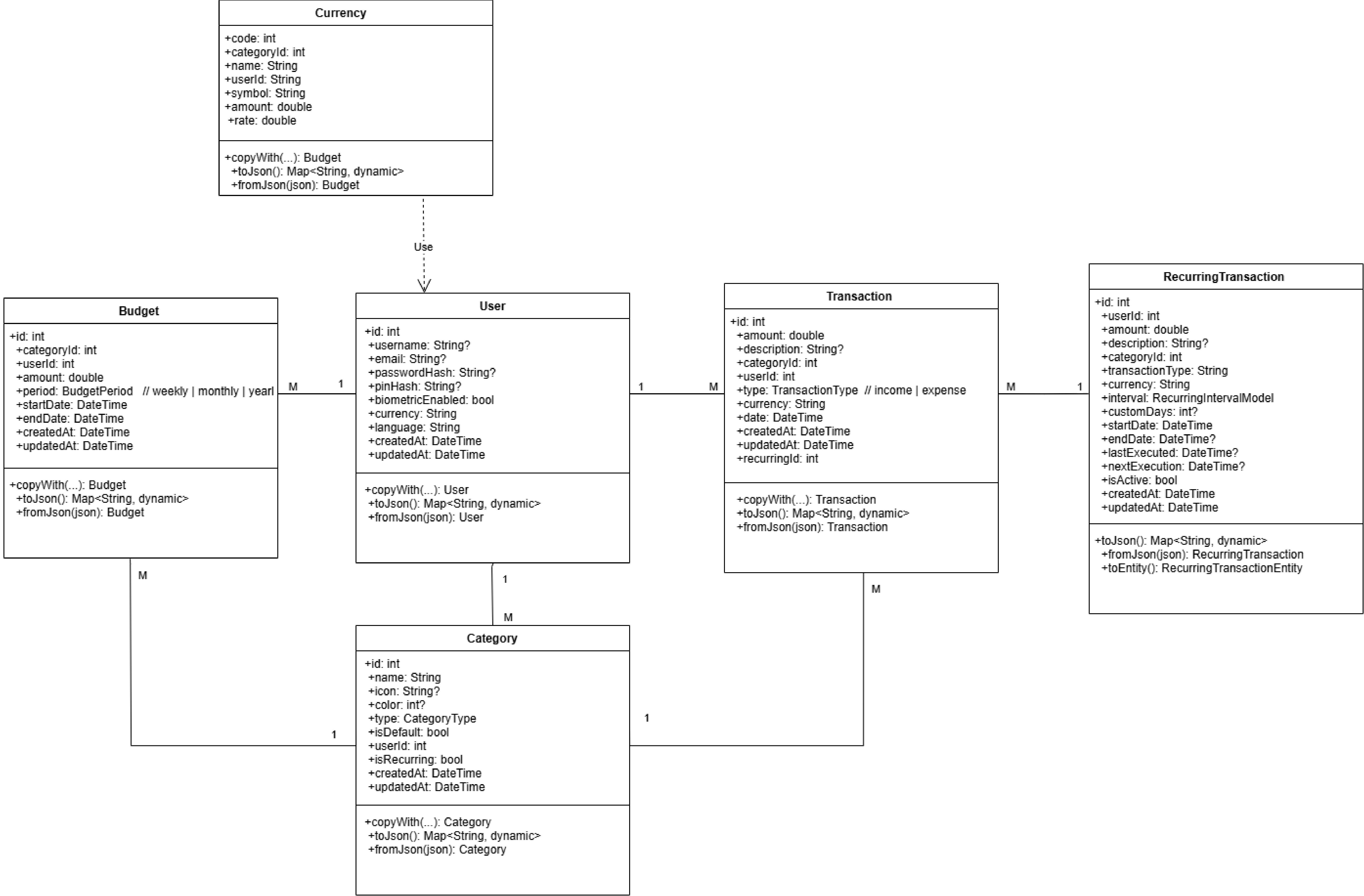
Диаграмма классов
