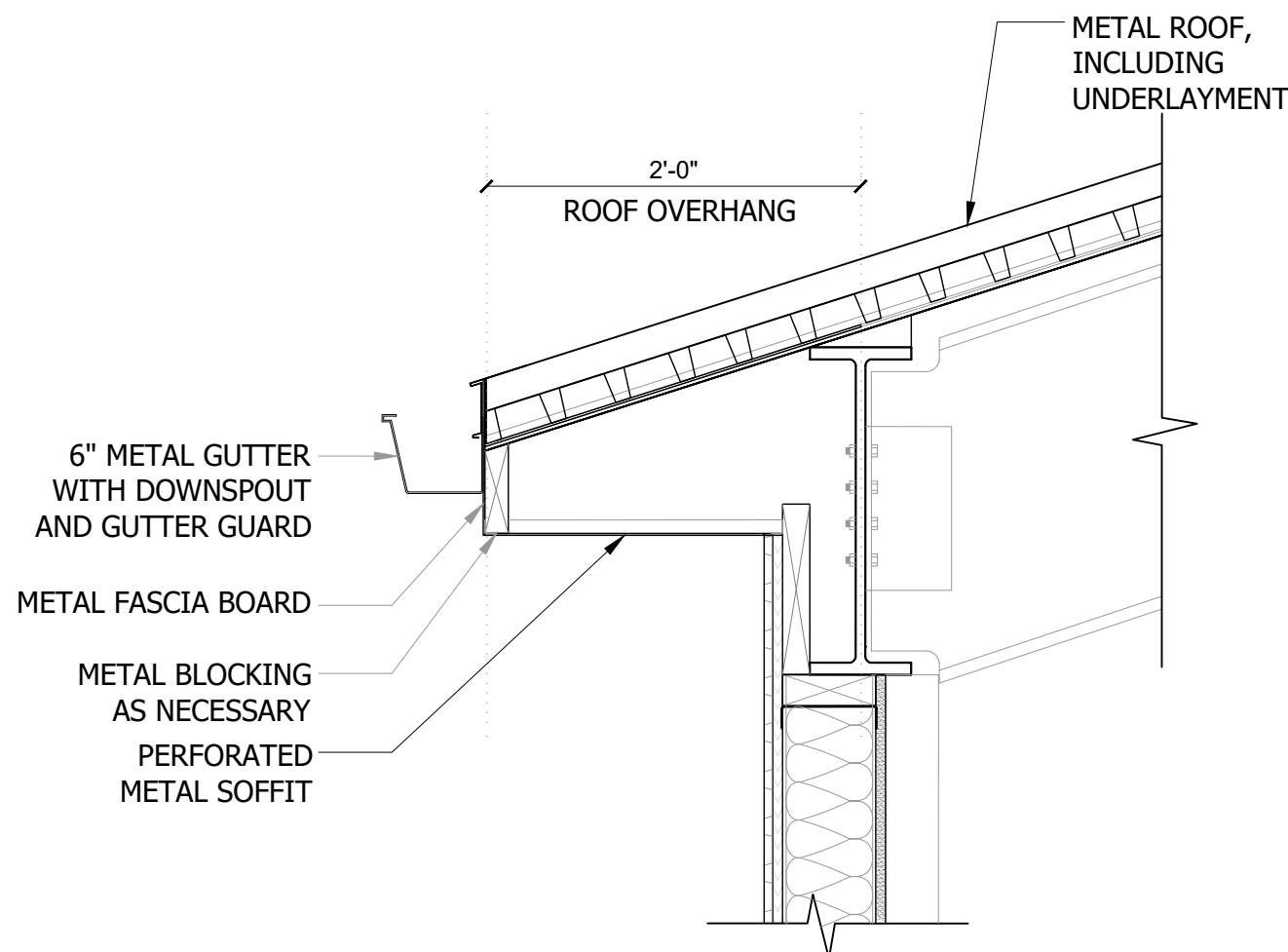
7 ROOF EDGE DETAIL C-303 SCALE: NTS
