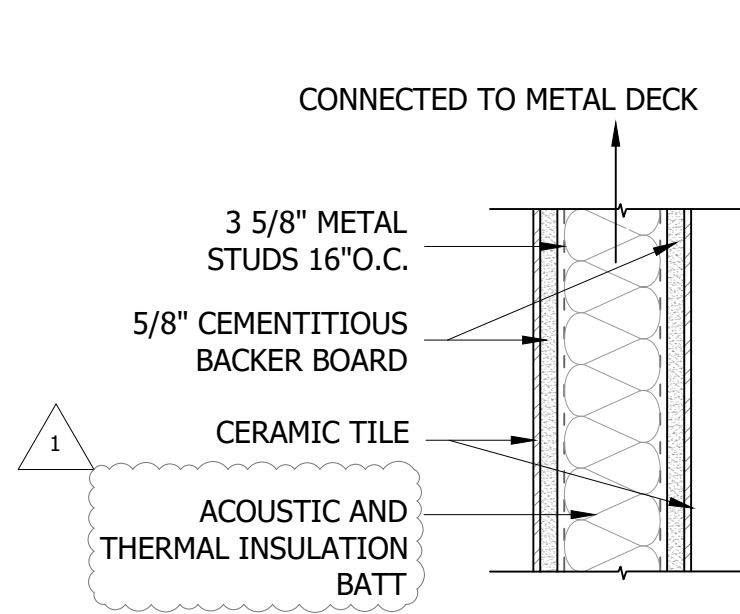
4" PARTITION WALL TYPE A1 SCALE: NTS
