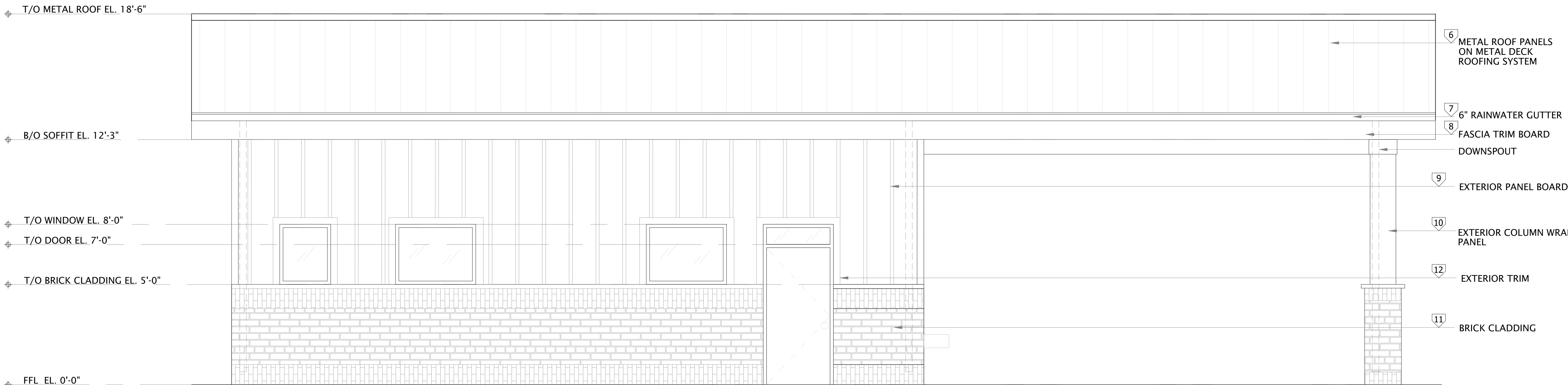
2 ELEVATION - C C-206 SCALE: 3/8" = 1'-0"
