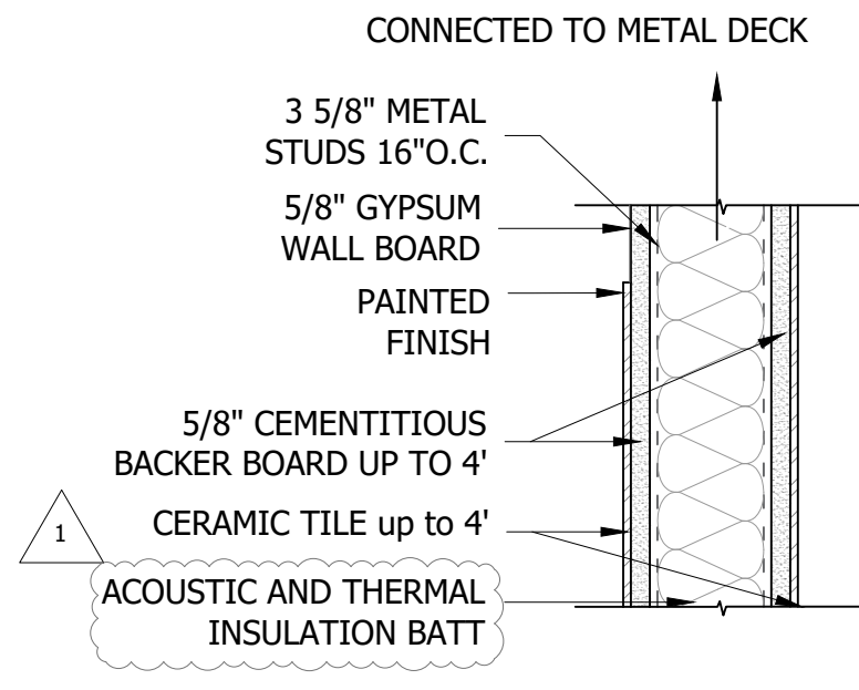
4" PARTITION WALL TYPE A3 SCALE: NTS
