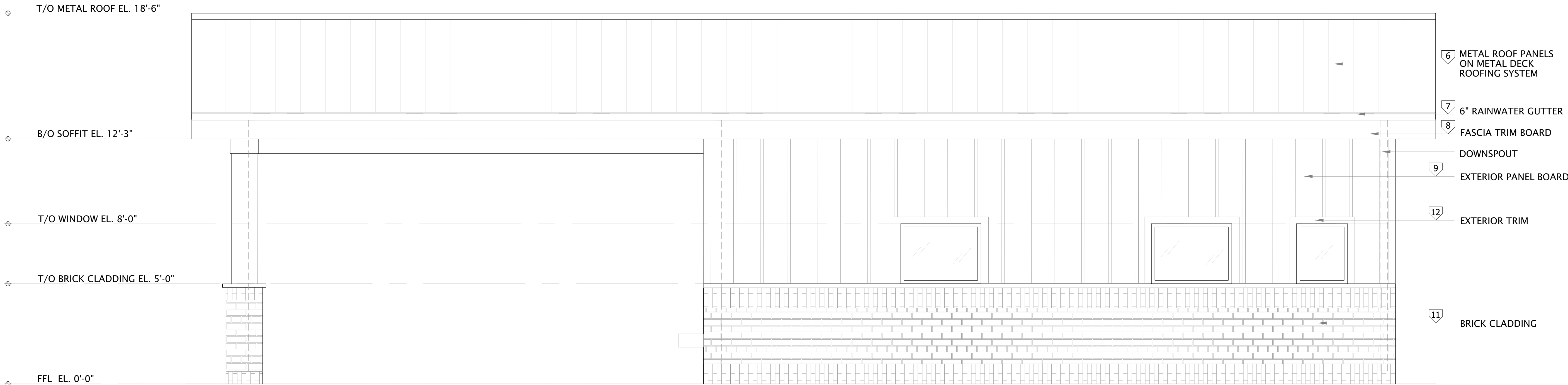
1 ELEVATION - A C-206 SCALE: 3/8" = 1'-0"
