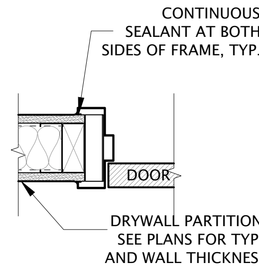
TYP. HM DOOR JAMB SCALE: NA
