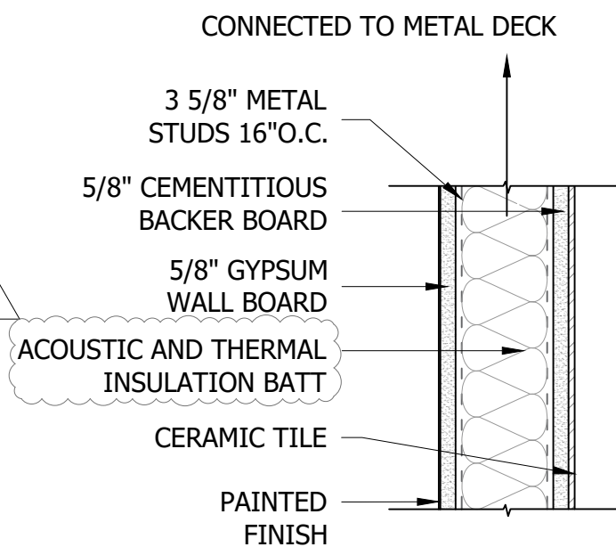
4" PARTITION WALL TYPE A2 SCALE: NTS
