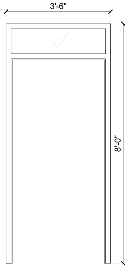
DOOR FRAME TYPE: DF2
