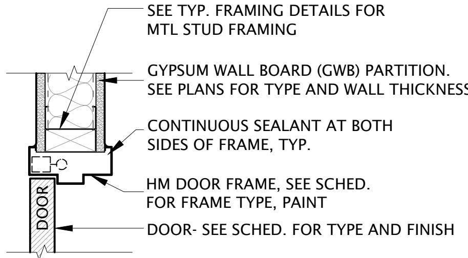
TYP. HM DOOR HEAD SCALE: NA
