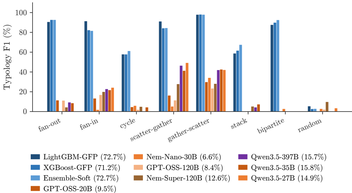
Per-class typology F1 on HI-Small
