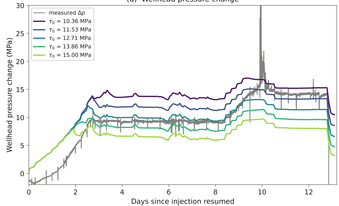
(d) Wellhead pressure change
