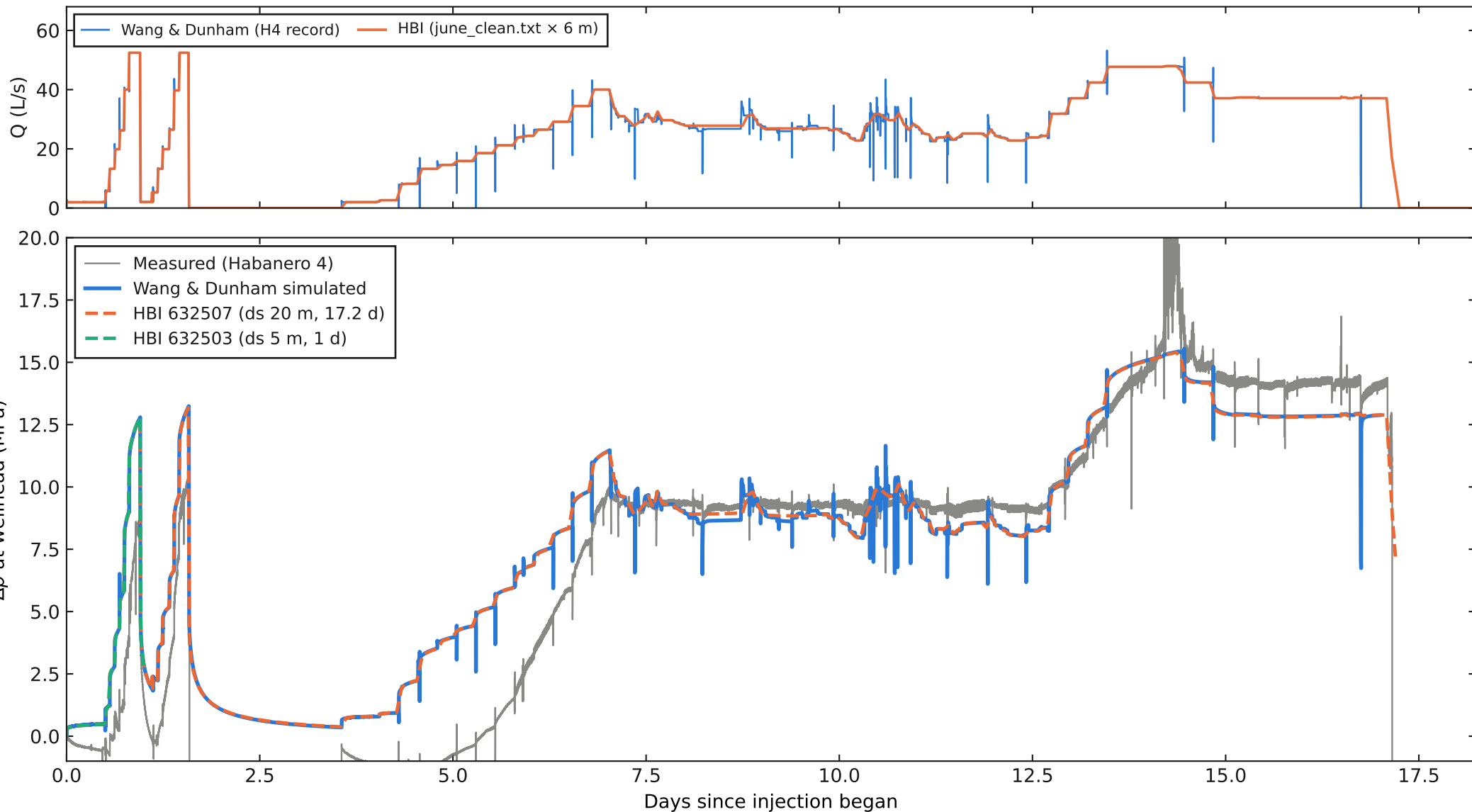
HBI vs Wang & Dunham (2022), Habanero 4
