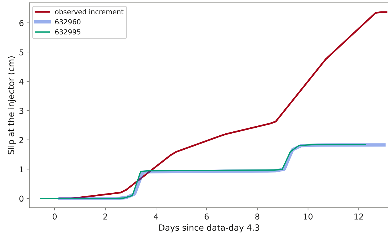
(d) Cumulative slip at the injector
