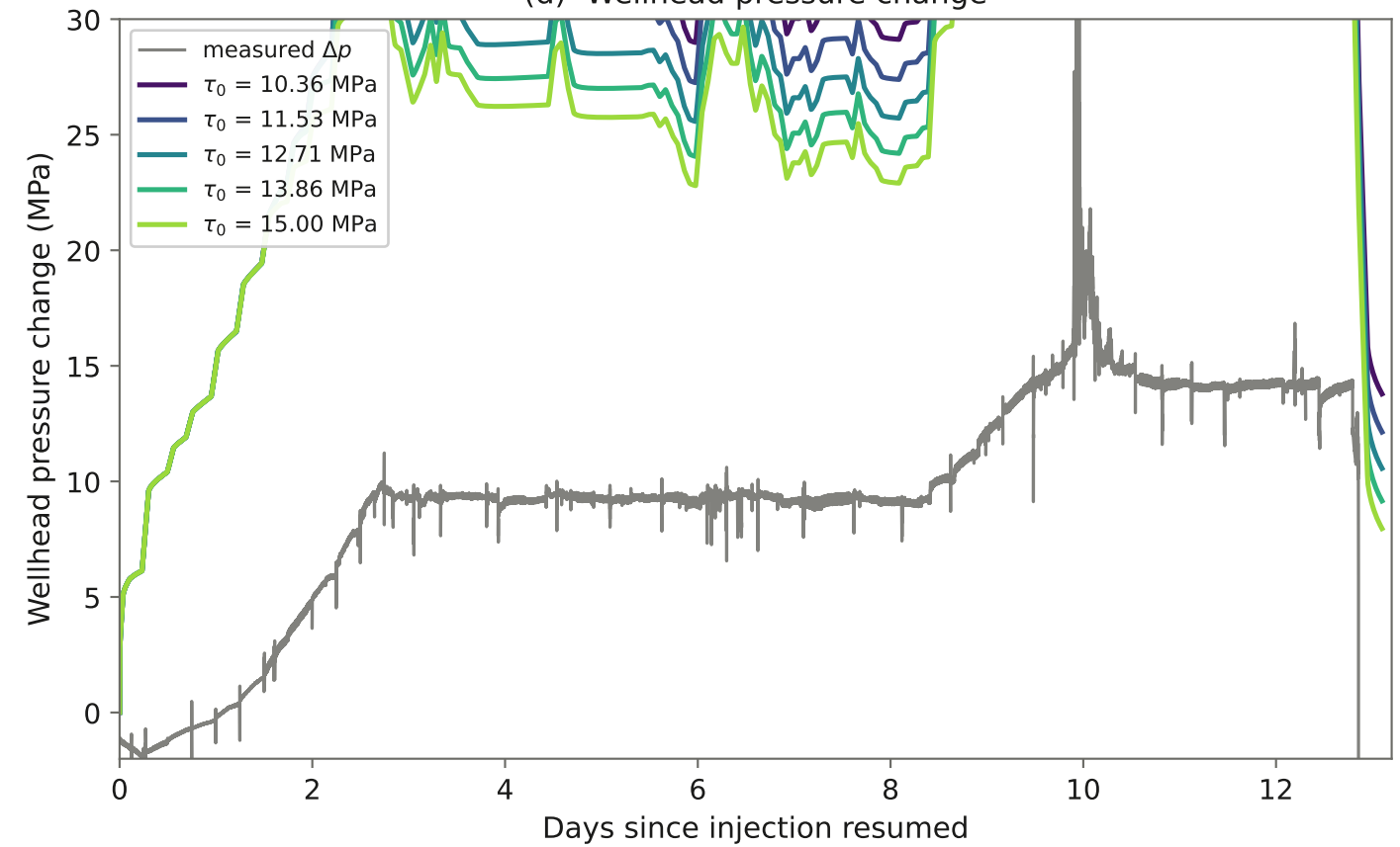
(d) Wellhead pressure change
