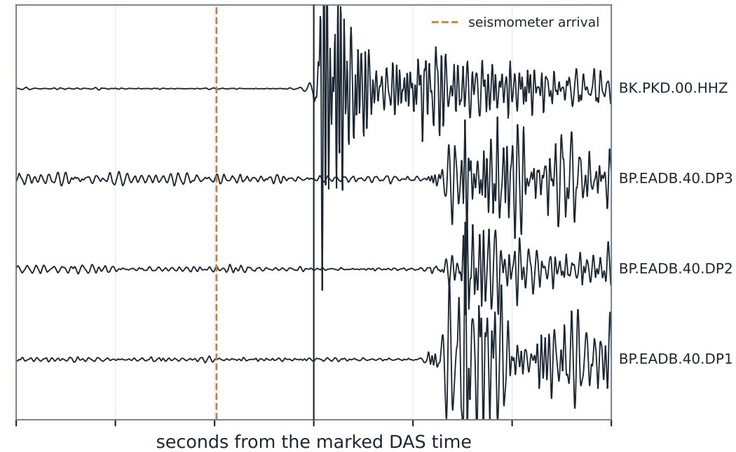
Seismometer recordings (5-20 Hz)
