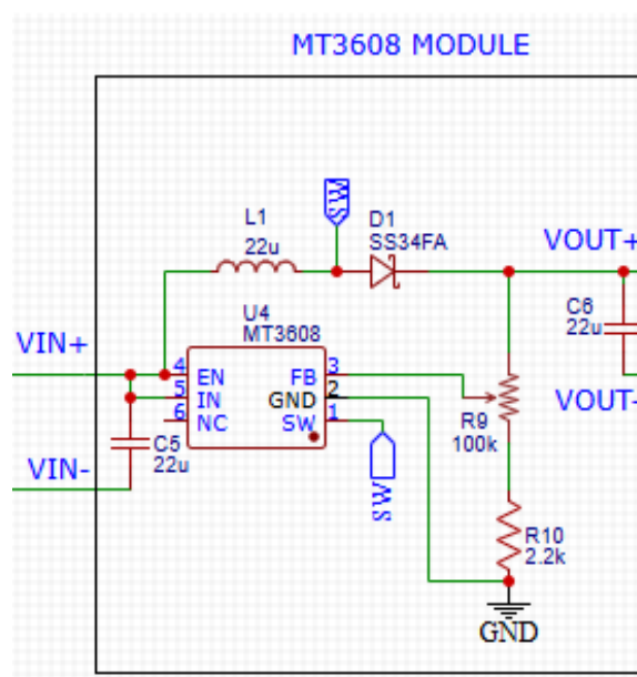
Figura 3.22: Circuito comercial de los módulos MT3608
