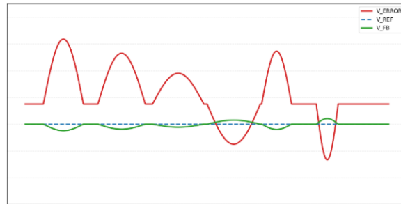
Figura 3.16: Gráfico explicativo del comportamiento del amplificador de error
