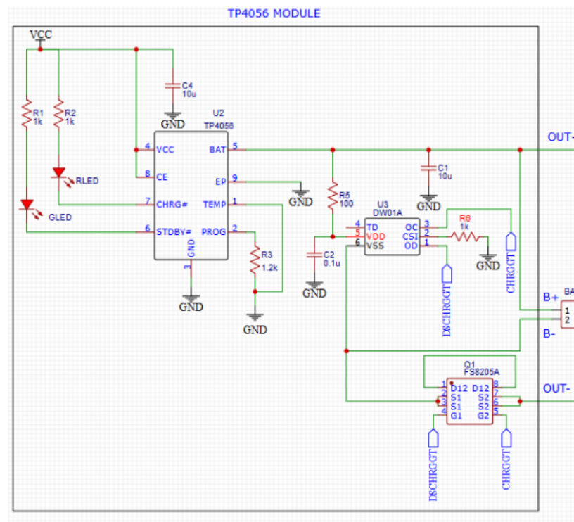
Figura 3.13: Circuito típico de aplicación del TP4056
