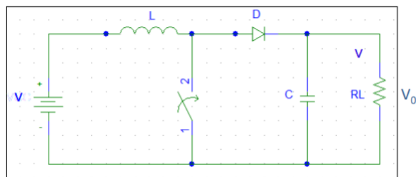
Figura 3.14: Circuito elevador Boost
