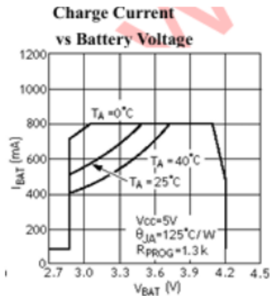
Figura 3.17: Corriente vs voltaje de carga
