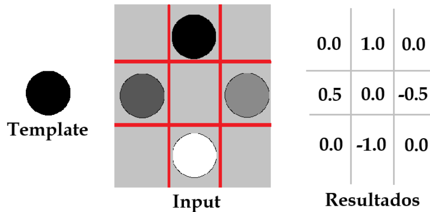
Figura 2.4: Imagen ilustrativa de una matriz de resultados de Template Matching
