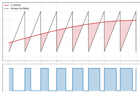
Figura 3.22: Modulación por ancho de pulso (PWM)
