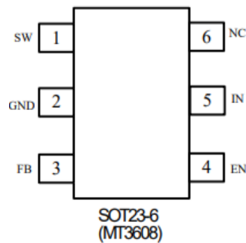
Figura 3.23: Diagrama de pines del módulo MT3608
