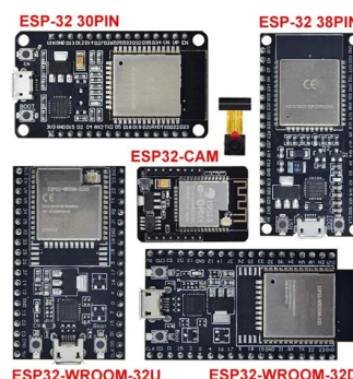
Figura 3.14: Algunas placas de desarrollo de la familia ESP32
