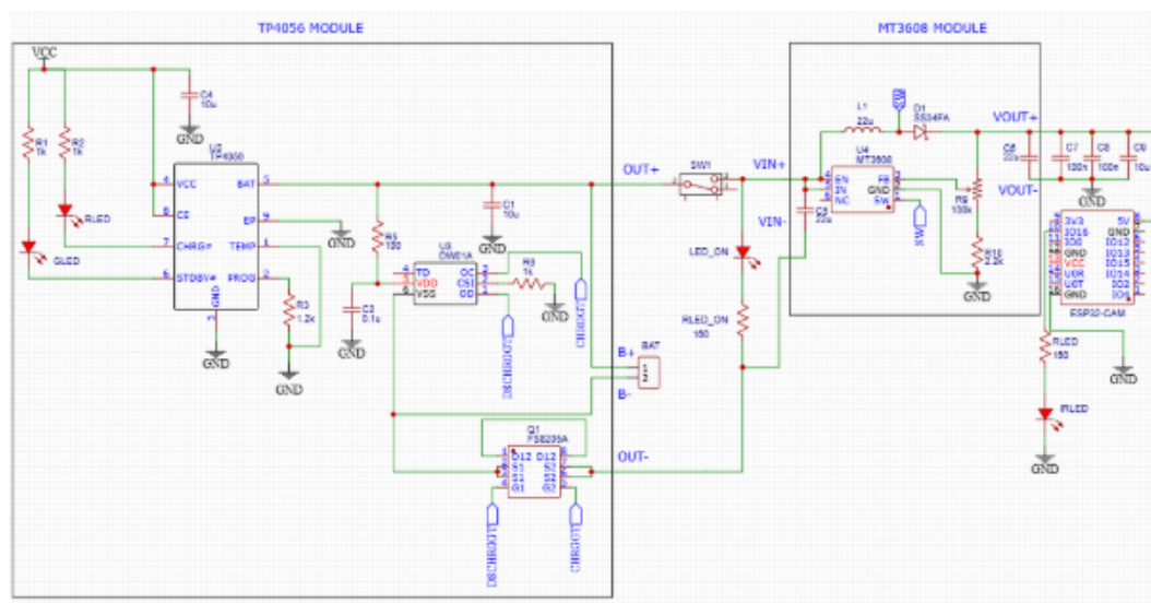
Figura 4.1: Esquema de conexiones para la PCB del circuito captador
