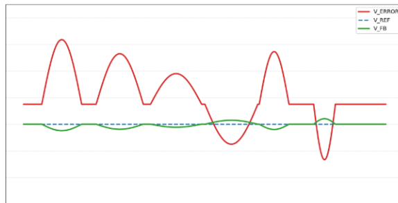
Figura 3.21: Gráfico explicativo del comportamiento del amplificador de error
