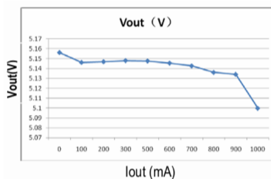
Figura 3.24: Regulación de carga del MT3608
