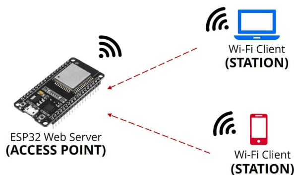
Figura 2.9: Red Wi-Fi con un microcontrolador ESP32 como punto de acceso
