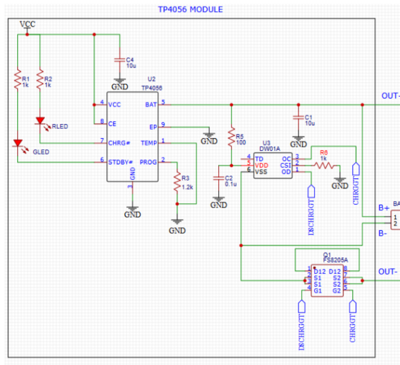
Figura 3.18: Circuito típico de aplicación del TP4056
