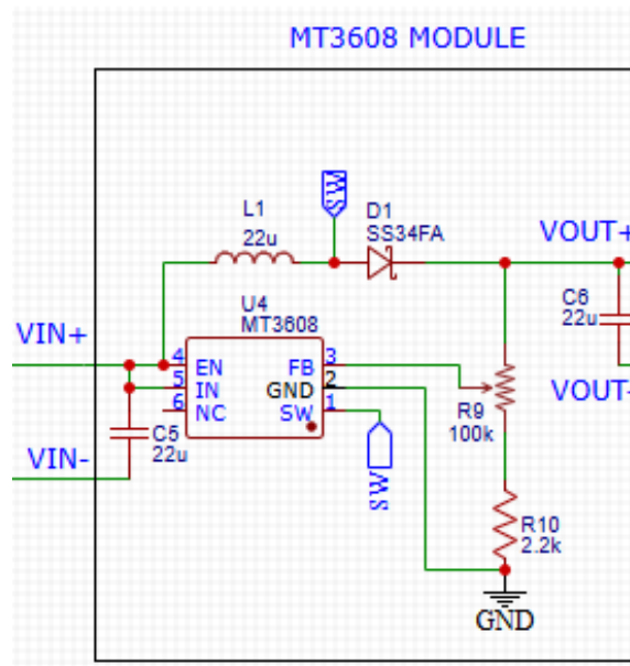
Figura 3.27: Circuito comercial de los módulos MT3608
