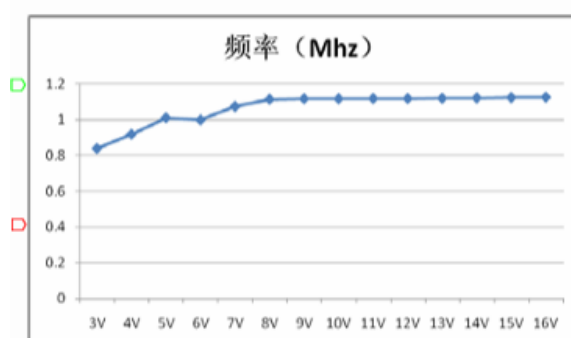
Figura 3.25: Frecuencia vs Tensión de entrada en el chip MT3608
