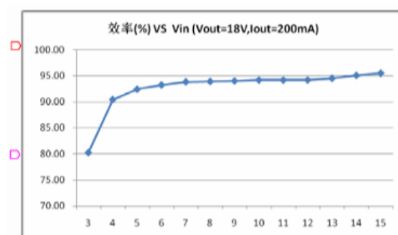
Figura 3.26: Eficiencia vs Tensión de entrada en el chip MT3608
