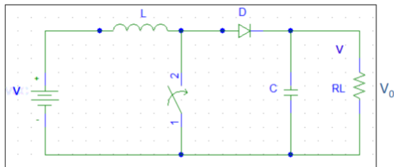
Figura 3.19: Circuito elevador Boost
