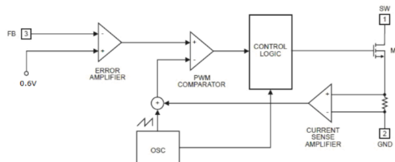
Figura 3.20: Circuito interno del chip MT3608
