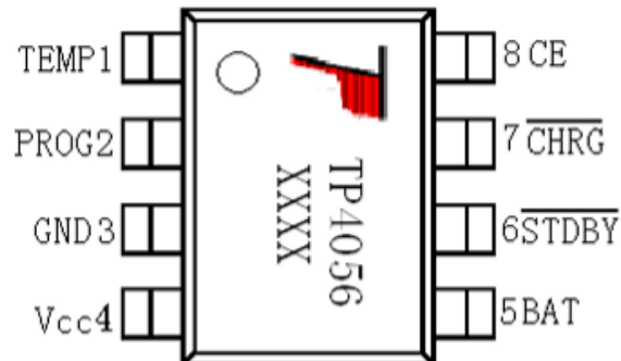
Figura 3.16: Diagrama de pines del módulo TP4056
