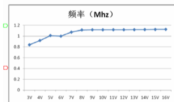
Figura 3.25: Frecuencia vs Tensión de entrada en el chip MT3608
