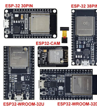
Figura 3.14: Algunas placas de desarrollo de la familia ESP32
