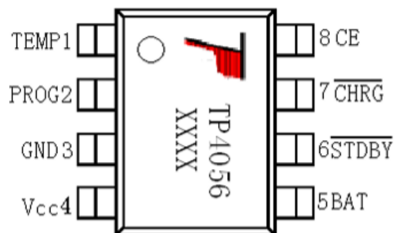
Figura 3.11: Diagrama de pines del módulo TP4056
