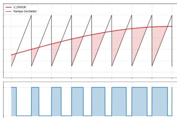
Figura 3.17: Modulación por ancho de pulso (PWM)
