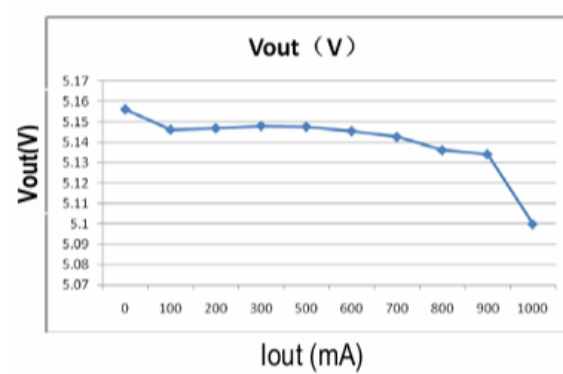
Figura 3.19: Regulación de carga del MT3608
