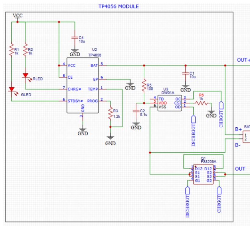
Figura 3.13: Circuito típico de aplicación del TP4056
