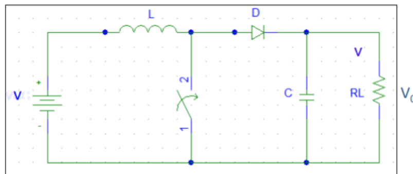
Figura 3.14: Circuito elevador Boost
