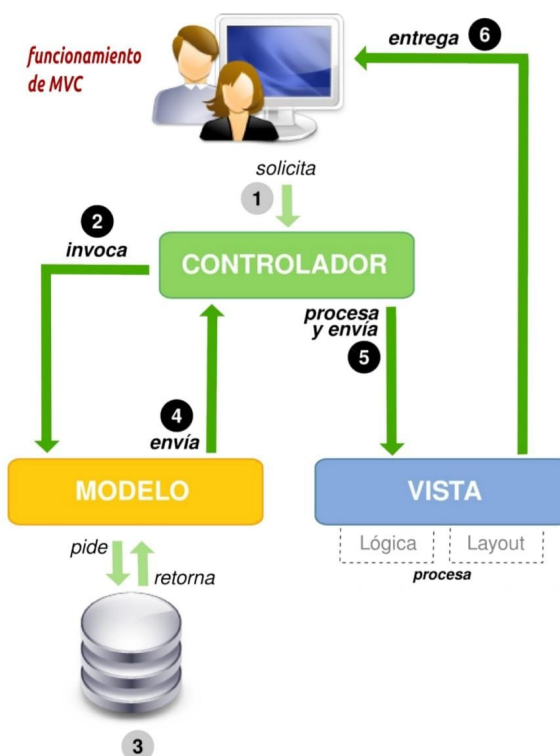
Figura 2.11: Patrón de diseño Modelo-Vista-Controlador (MVC)
