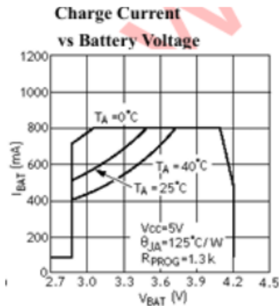
Figura 3.12: Corriente vs voltaje de carga
