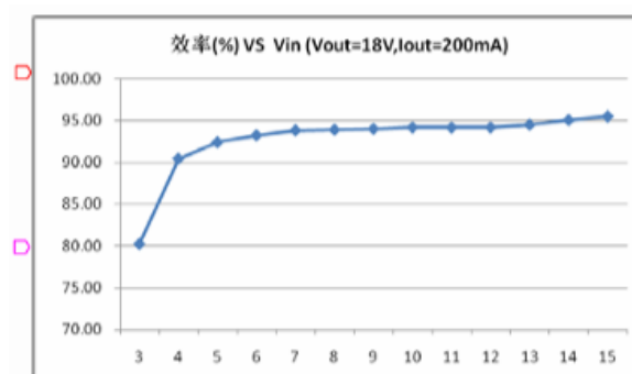
Figura 3.21: Eficiencia vs Tensión de entrada en el chip MT3608
