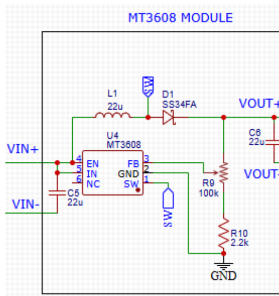
Figura 3.22: Circuito comercial de los módulos MT3608
