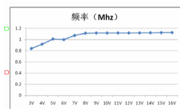
Figura 3.20: Frecuencia vs Tensión de entrada en el chip MT3608
