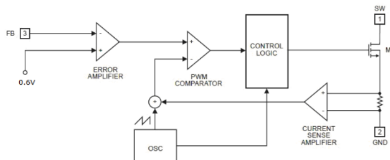
Figura 3.15: Circuito interno del chip MT3608
