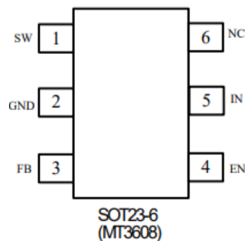
Figura 3.18: Diagrama de pines del módulo MT3608
