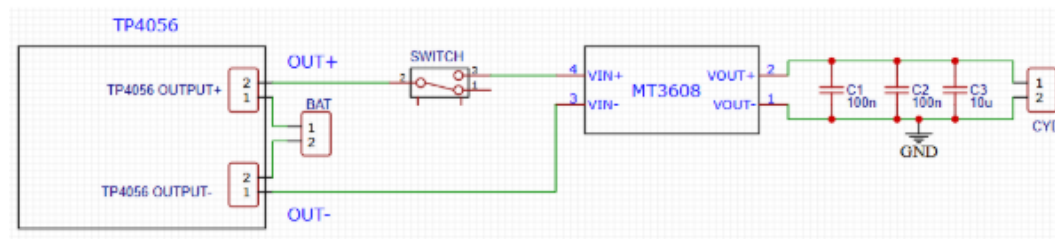
Figura 4.3: Esquema simplificado de la PCB del circuito servidor
