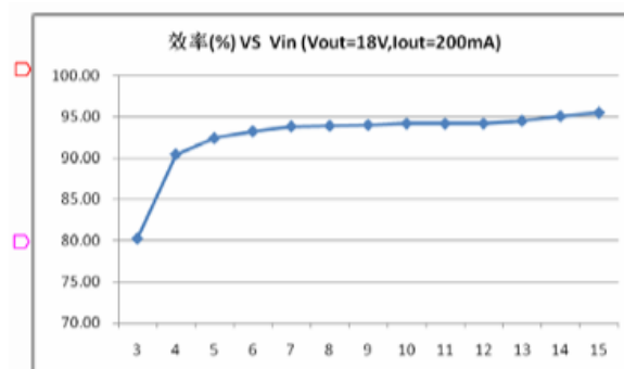
Figura 3.28: Eficiencia vs Tensión de entrada en el chip MT3608
