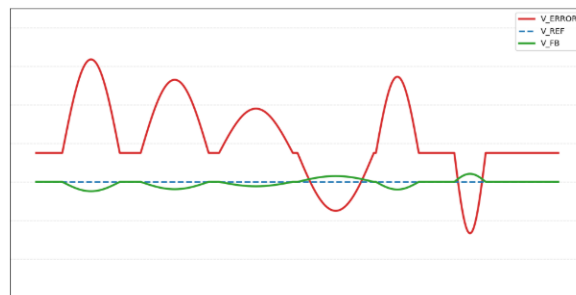
Figura 3.23: Gráfico explicativo del comportamiento del amplificador de error
