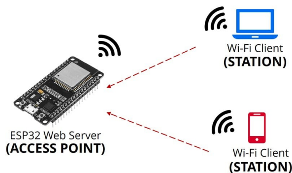
Figura 2.6: Red Wi-Fi con un microcontrolador ESP32 como punto de acceso
