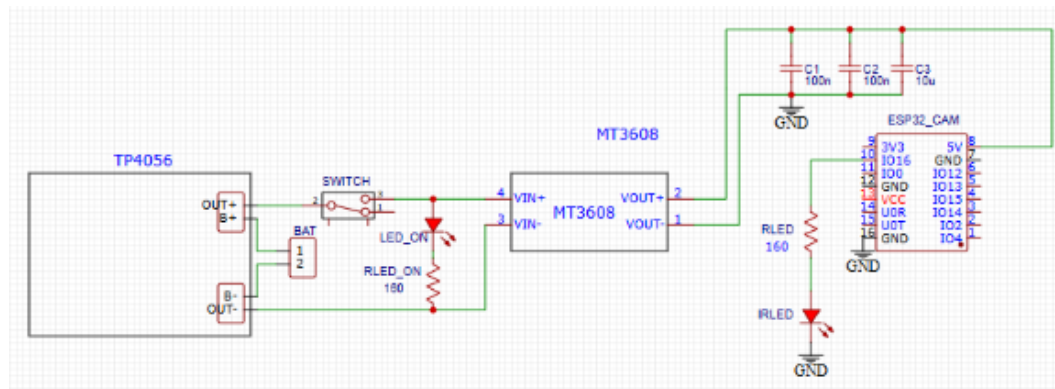
Figura 4.2: Esquema simplificado de la PCB del circuito captador
