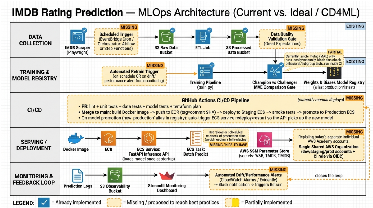
Figura 9: Arquitectura ideal propuesta (CD4ML): componentes ya implementados versus componentes faltantes para una solución MLOps completa.
