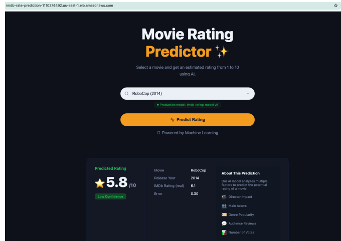
Figura 8: Ejemplo de predicción - Robocop(2014)
