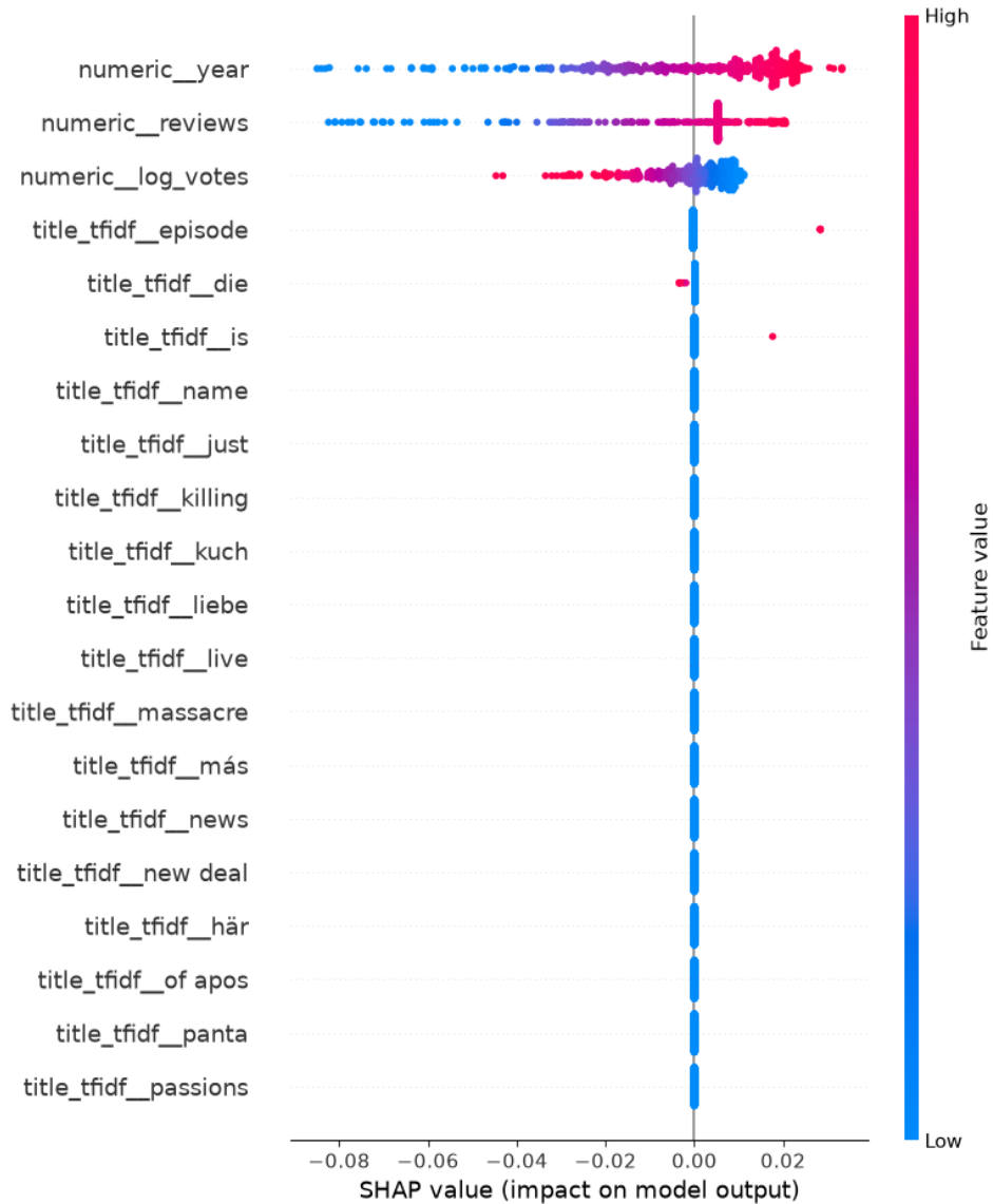
Figura 4: SHAP summary plot con las 20 features más influyentes en las predicciones sobre el test set.
