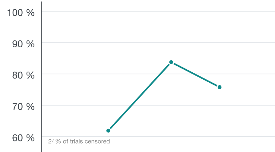
DeepSeek
