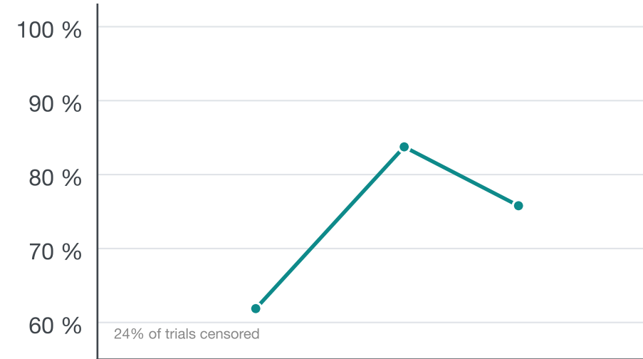
DeepSeek
