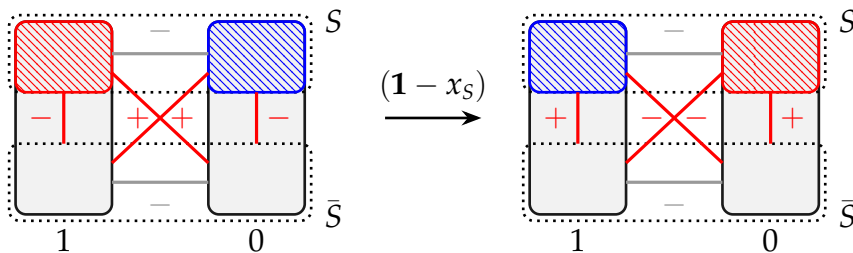
Fig. Correspondência de soluções.
