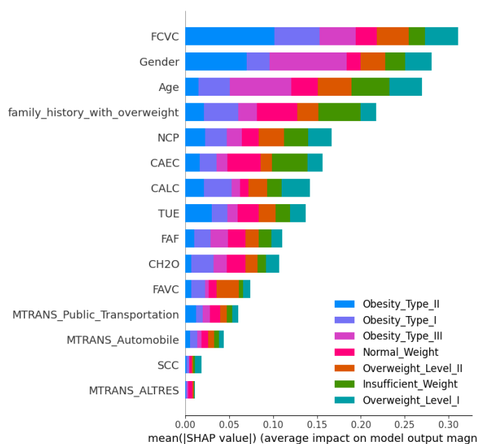
Figure 8. Gràfic de barres amb el pes de cada variable del model
