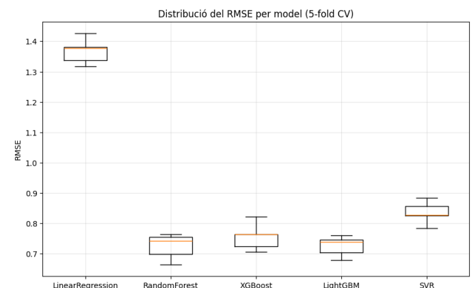
Figure 2. Visualització dels rangs dels RMSE dels algorismes
