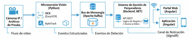
Diagrama de Componentes: Interacción de Módulos
