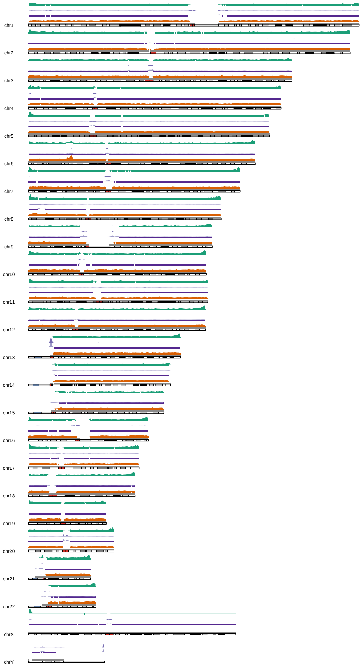
HG002 Q100 Variant Benchmark
