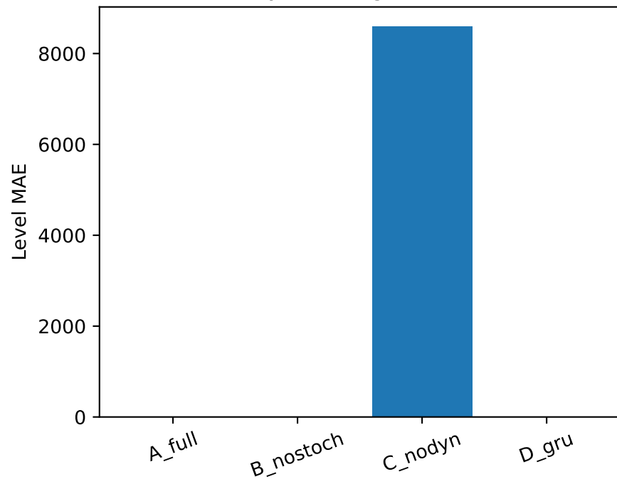
Horizon 1y (val targets 2016-2020)
