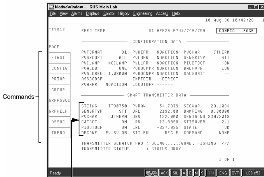
Transmitter Parameters
