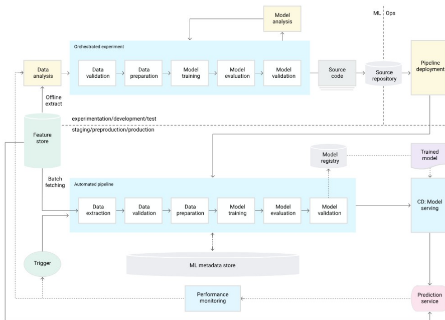
Gambar II.2 MLOps level 1 : otomatisasi training pipeline dengan komponen yang dapat dipakai ulang (Google Cloud 2024).
