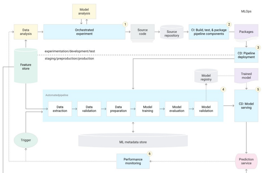
Gambar II.3 MLOps level 2 : orkestrasi CI/CD/CT dengan deteksi drift sebagai pemicu retraining (Google Cloud 2024).
