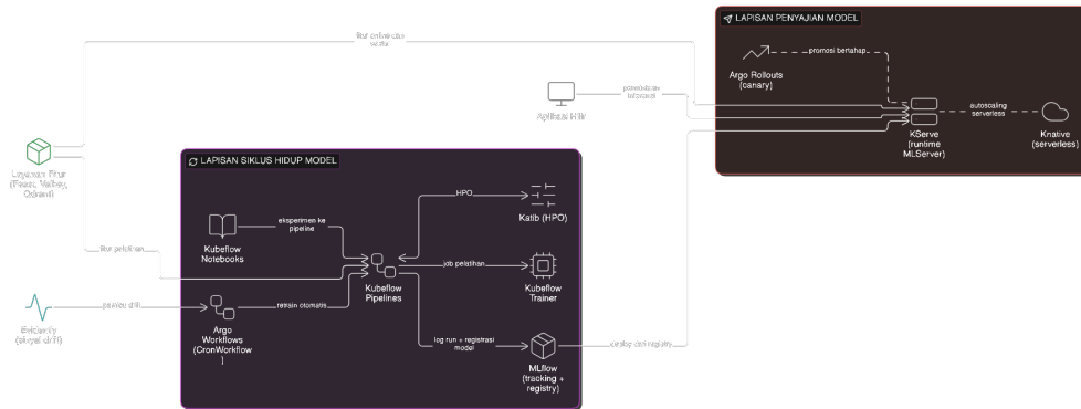
Gambar IV.4 Rincian Lapisan Siklus Hidup Model dan Penyajian
