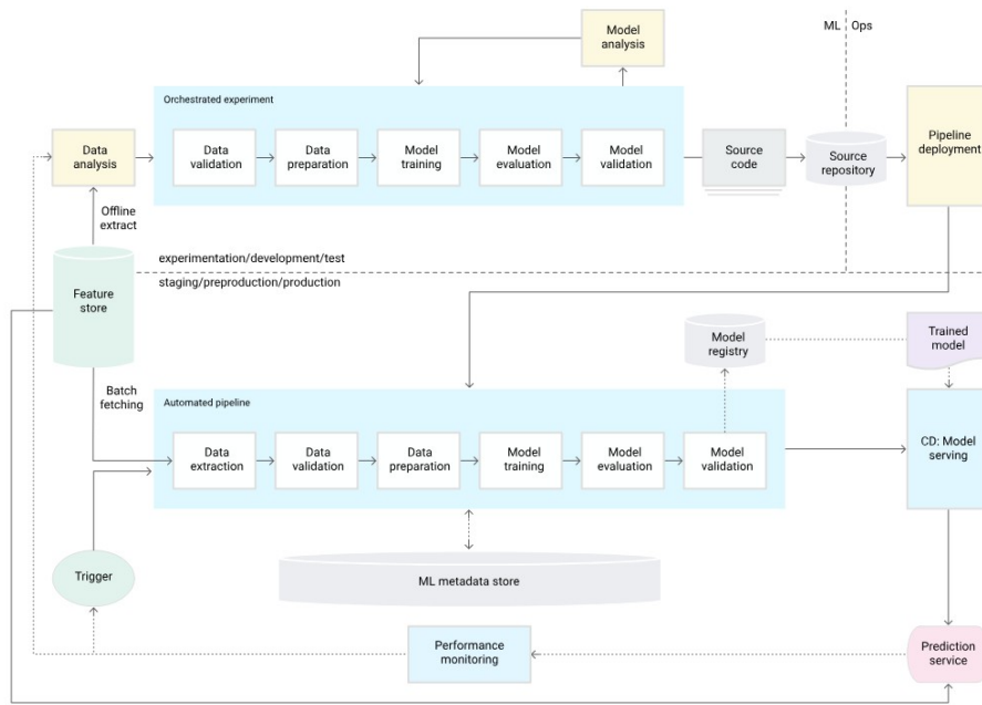
Gambar II.2 MLOps level 1 : otomasi training pipeline dengan komponen yang dapat dipakai ulang (Google Cloud 2024).
