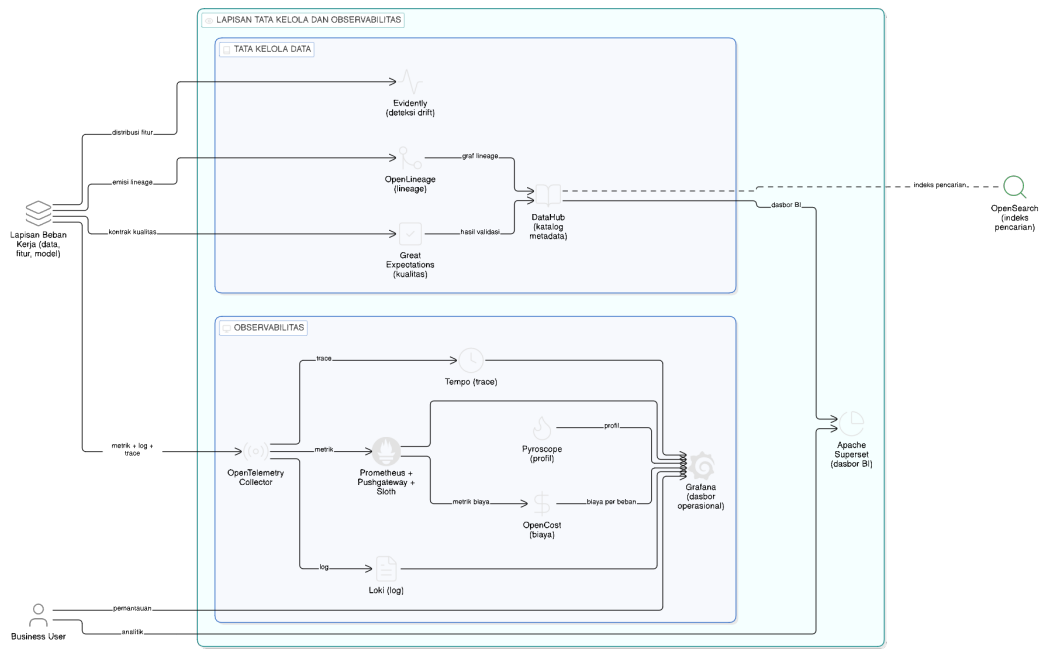
Gambar IV.19 Rincian bagian observabilitas pada Governance and Observability Layer
