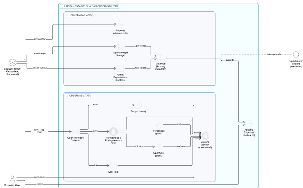
Gambar IV.18 Rincian bagian tata kelola data pada Governance and Observability Layer
